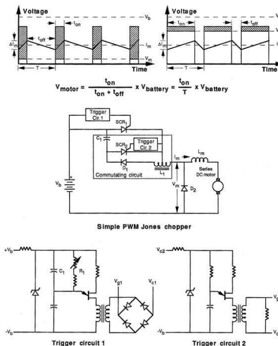
Gambar 7.1 Ringkasan Karakteristik Kontroler Helikopter PWM sakelar Jones.
