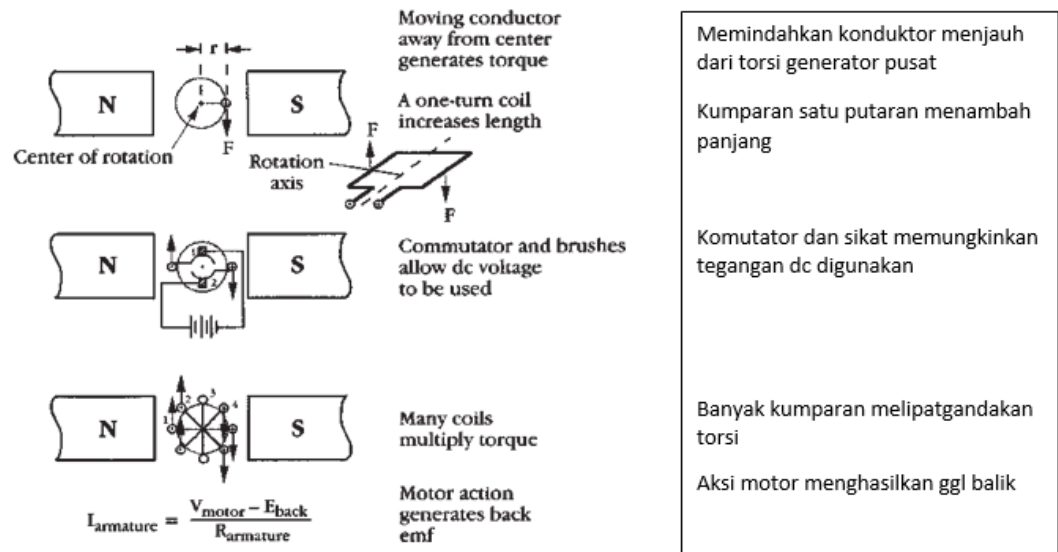
Gambar 6.2 Dasar-dasar motor DC, mendapatkan torsi dari konduktor yang bergerak.
