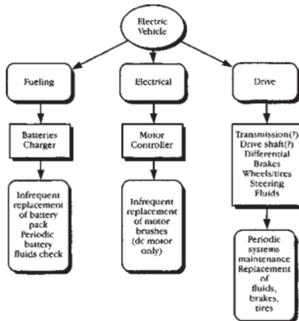
Gambar 1.4 Sistem kendaraan listrik.
