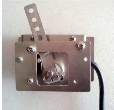
Gambar 9.8 Potensiometer throttle Curtis dengan sakelar penonaktifan pedal tinggi (perhatikan tiga kontak sakelar di sebelah kiri).
