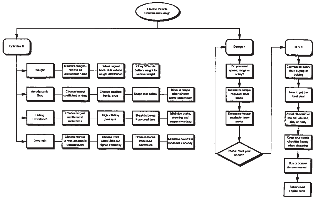
Gambar 5.1 Pentingnya Meminimalkan Bobot Di Mobil Listrik
