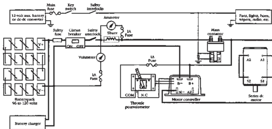
Gambar 9.6 Diagram Pengkabelan Dasar Kendaraan Listrik.
