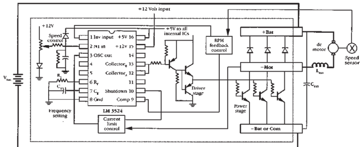
Gambar 7.2 Desain pengontrol nyata menggunakan LM3524.
