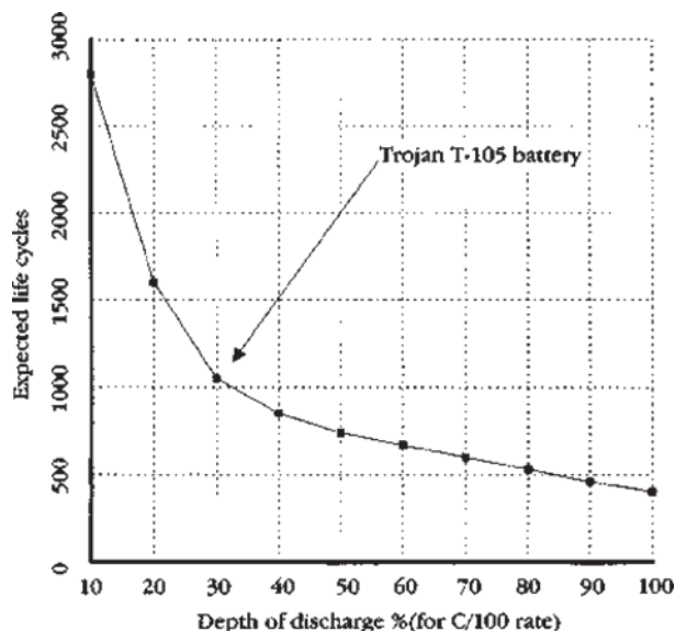
Gambar 8.7 Kedalaman debit versus siklus hidup yang diharapkan untuk baterai Trojan T-105 y.
