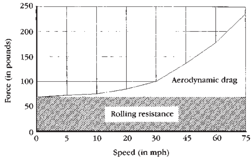
Gambar 5.5 Resistensi rolling dan drag aerodinamis dibandingkan kecepatan.
