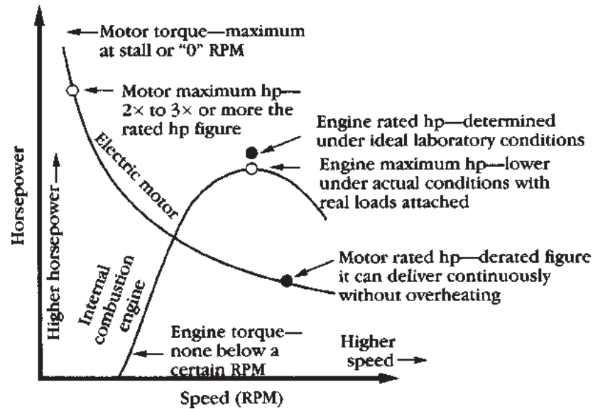
Gambar 5.7 Perbandingan Motor Listrik Dengan Karakteristik Mesin Pembakaran Dalam.
