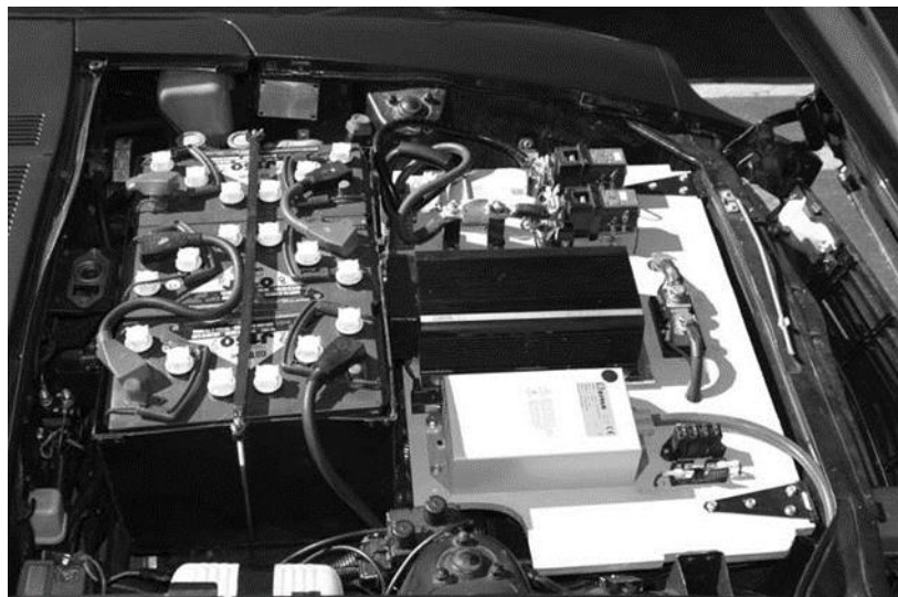
Gambar 10.14 Baterai Operasi Z terpasang pada tempatnya.
