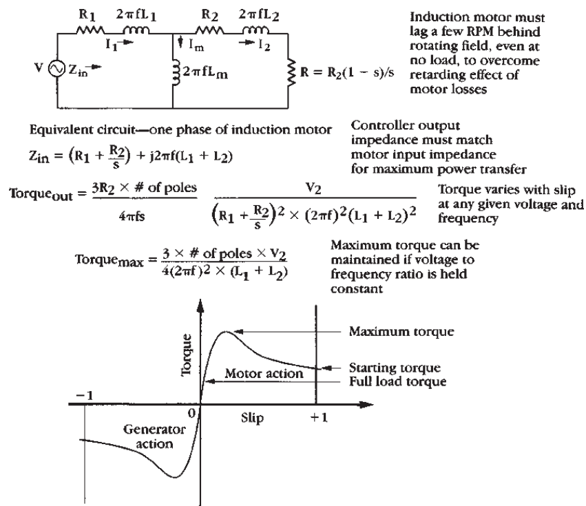
Gambar 6.9 Karakteristik kecepatan, torsi, dan slip unik motor AC polifase versus tegangan dan frekuensi.
