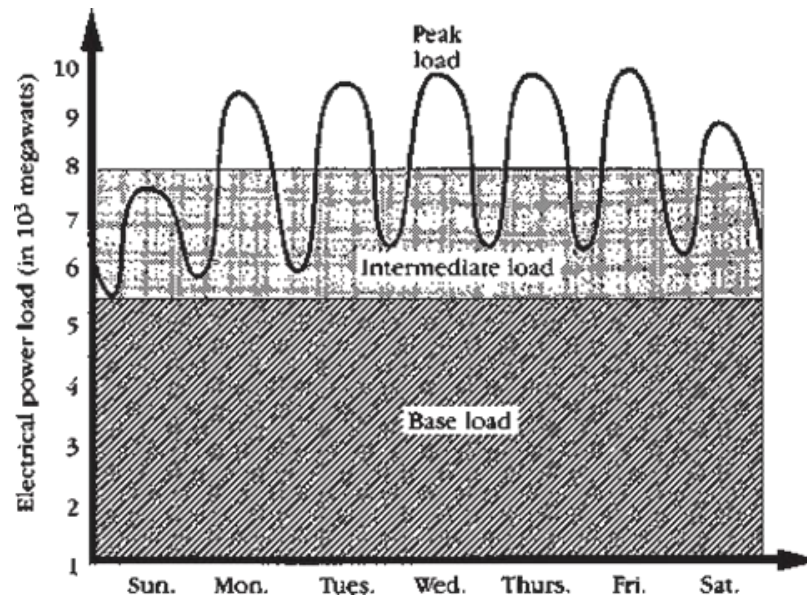
Gambar 2.4 Kurva permintaan daya puncak mingguan untuk utilitas besar yang beroperasi dengan faktor beban mingguan sekitar 80%.
