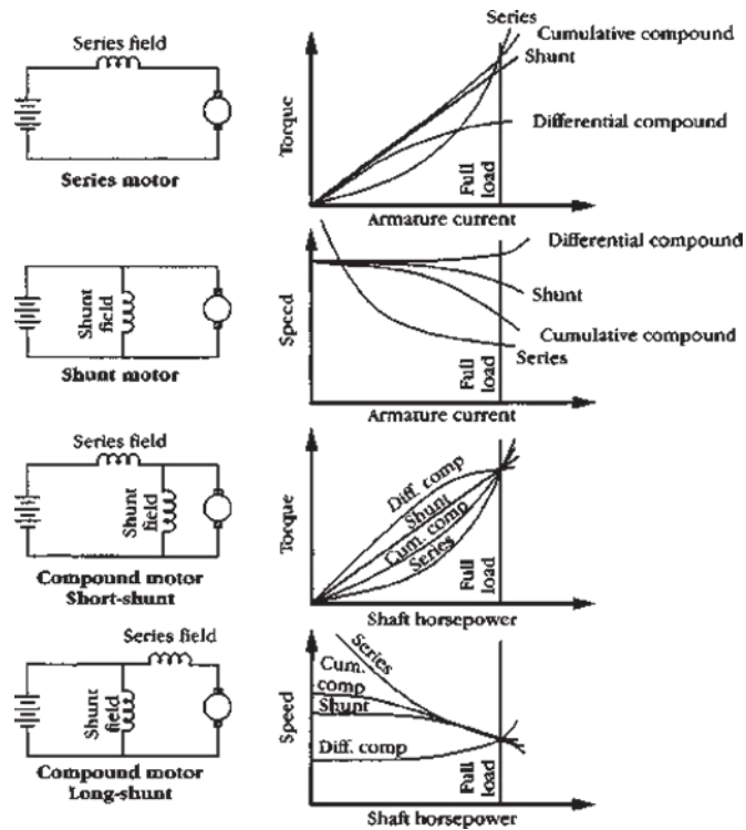
Gambar 6.3 Ringkasan jenis motor DC
