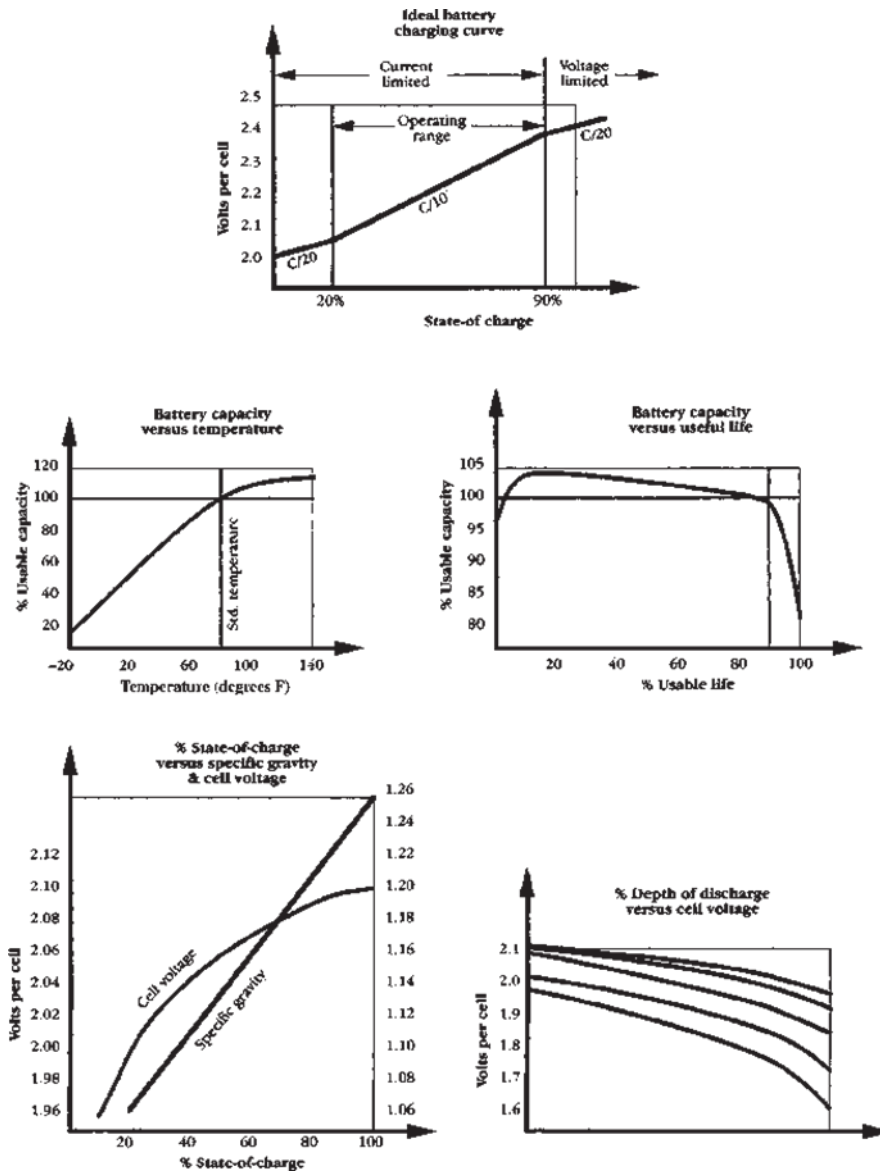
Gambar 8.2 Karakteristik Pengisian Dan Pengosongan Baterai Timbal-Asam.
