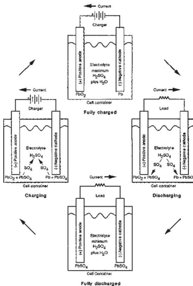
Gambar 8.1 Kimia Sel Timbal-Asam Sederhana.
