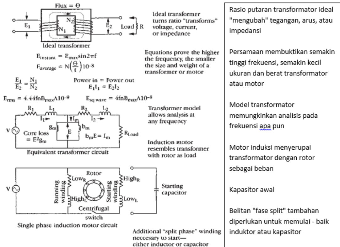
Gambar 6.7 Motor AC menyerupai transformator.
