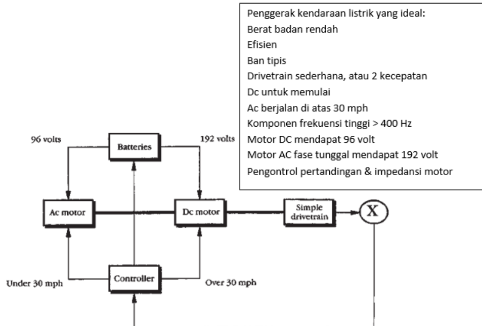
Gambar 6.15 Solusi motor kendaraan listrik terbaik di masa depan.
