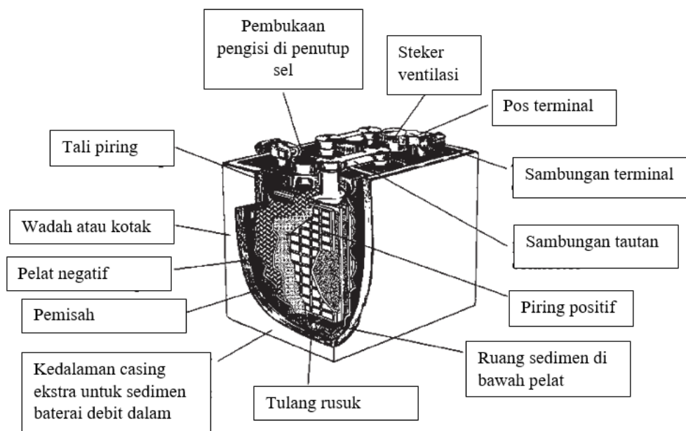
Gambar 8.3 Konstruksi Baterai Timbal-Asam.
