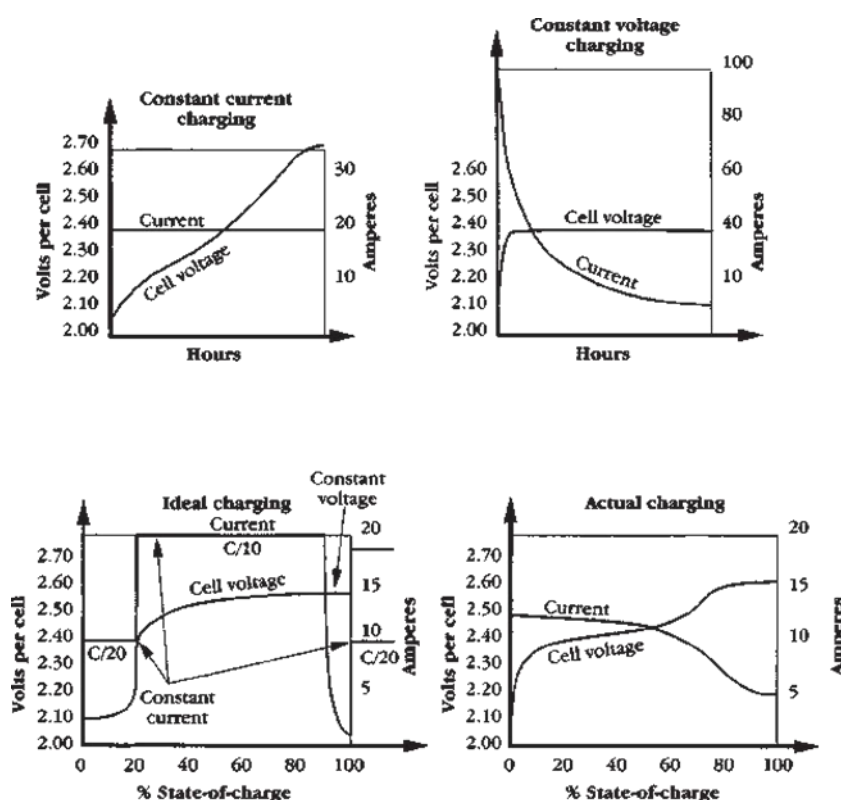
Gambar 9.3 Karakteristik Pengisian Baterai Timbal-Asam Yang Ideal Dan Aktual.
