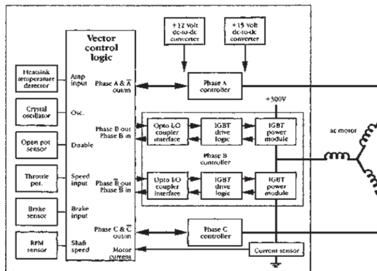
Gambar 7.4 Tujuan perancangan pengontrol AC dan diagram blok.
