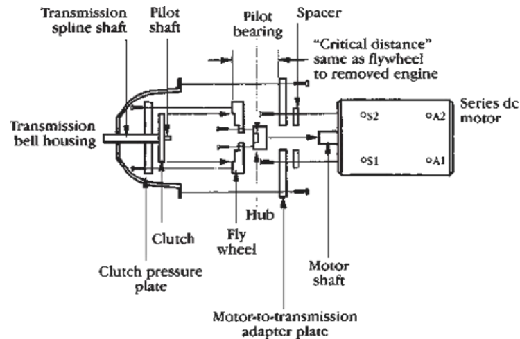
Gambar 10.8 Elemen Motor Listrik Ke Proses Penyambungan Transmisi Mekanis.
