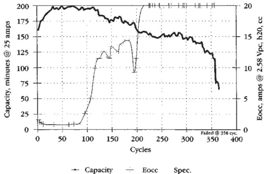
Gambar 9.1 Hasil Uji Siklus Hidup Untuk Baterai Asam Timbal Siklus Dalam Trojan 27TMH y.
