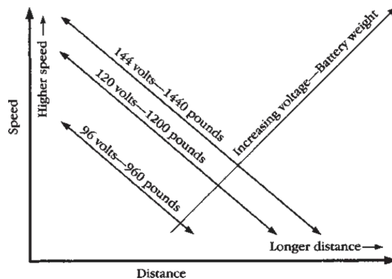
Gambar 4.14 Lebih banyak baterai selalu lebih baik daripada lebih sedikit sampai titik tertentu.
