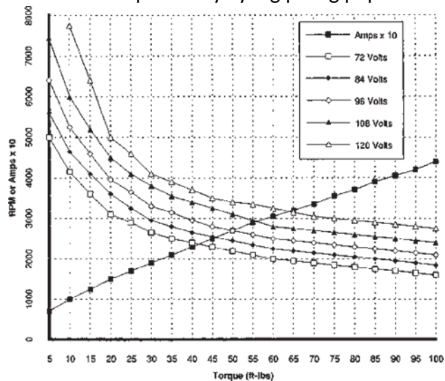
Gambar 6.14 Kecepatan dan arus motor DC seri FB1-4001 lanjutan versus kurva torsi.
