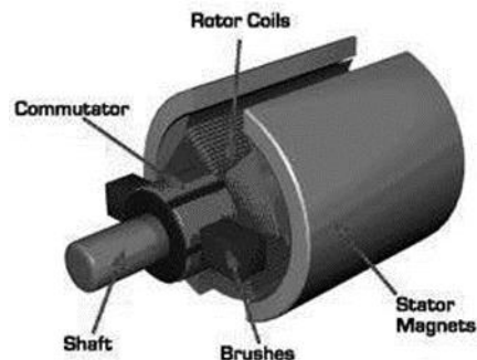
Gambar 6.4 Motor DC magnet permanen (Uji coba kendaraan Nol Emisi Australia dan www.mobil-listrik-untuk-anak-perempuan.com ).
