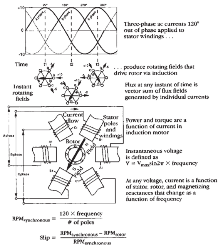
Gambar 6.8 Operasi motor polifase AC diringkas.
