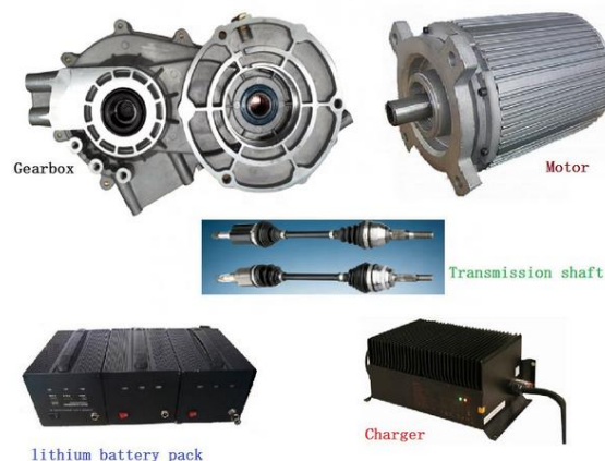
Gambar 10.7 Kit kendaraan listrik.
