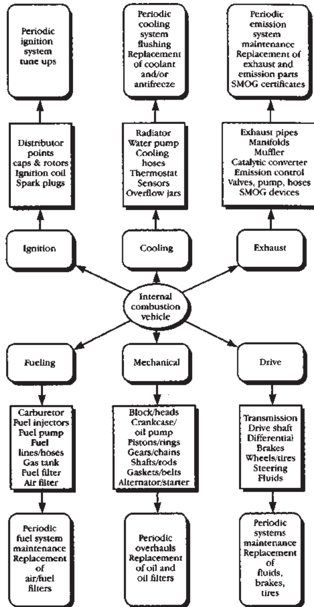
Gambar 1.3 Sistem mesin pembakaran dalam.
