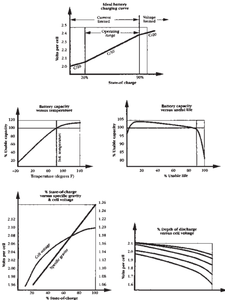
Gambar 9.2 Rangkuman Grafis Dari Siklus Pengosongan Dan Pengisian Baterai.
