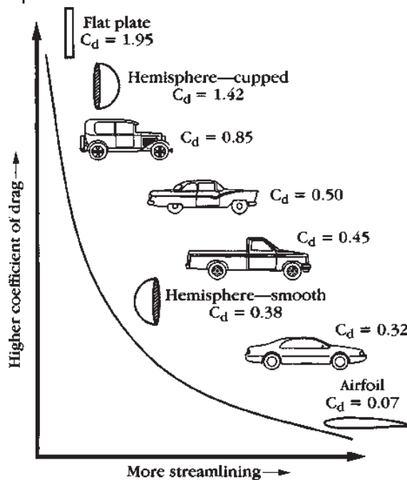
Gambar 5.4 Koefisien Ringkasan Drag Untuk Jenis Kendaraan Yang Berbeda.
