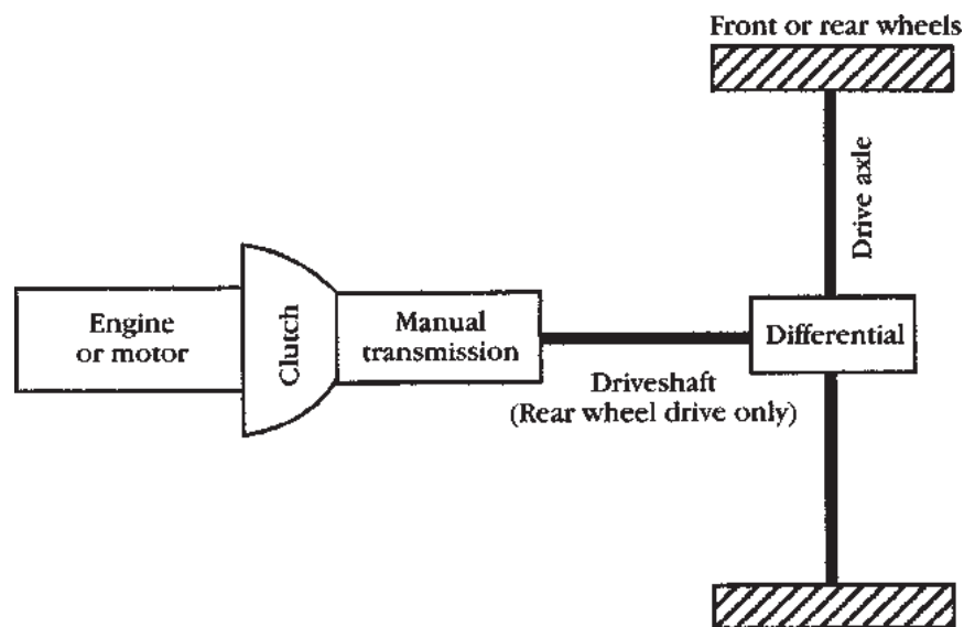
Gambar 5.6 Tata letak drivetrain motor listrik yang disederhanakan.
