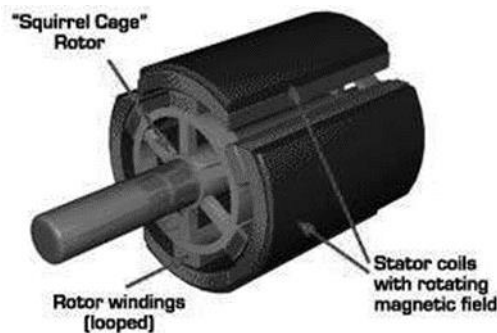
Gambar 6.10 Motor listrik AC (Uji Jalan Kendaraan Nol Emisi Australia).
