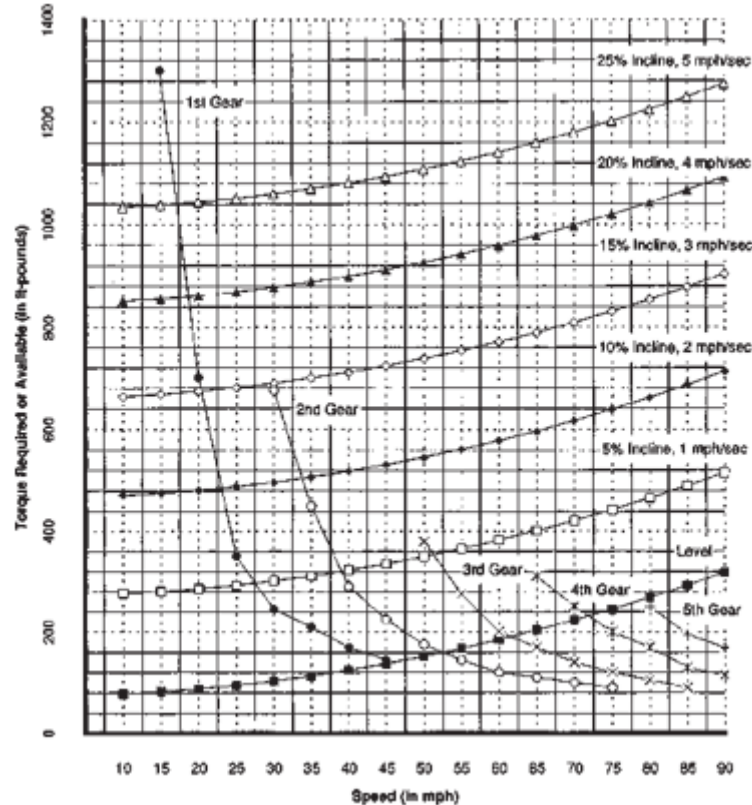
Gambar 5.9 Torsi Kendaraan Listrik Diperlukan Versus Torsi Yang Tersedia.
