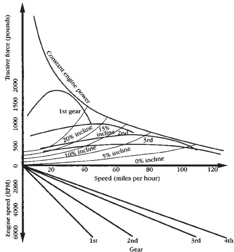
Gambar 5.8 Rasio gigi transmisi versus kecepatan dan ringkasan daya.
