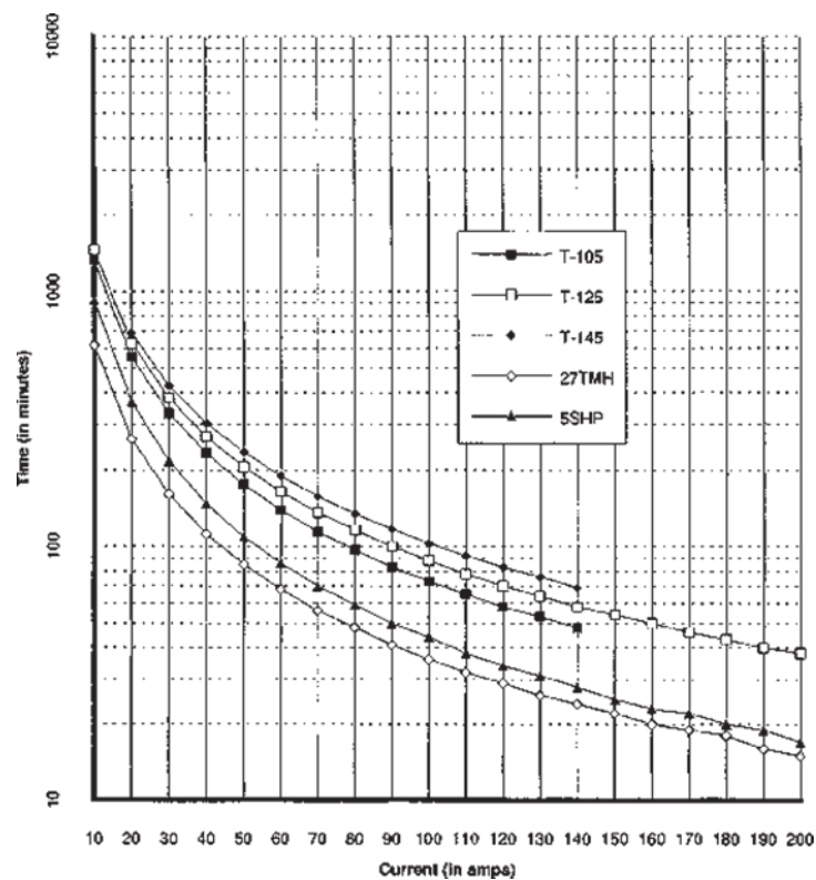
Gambar 8.6 Baterai siklus-dalam Trojan 6-volt dan 12-volt waktu keluarga versus kurva sewa saat ini.
