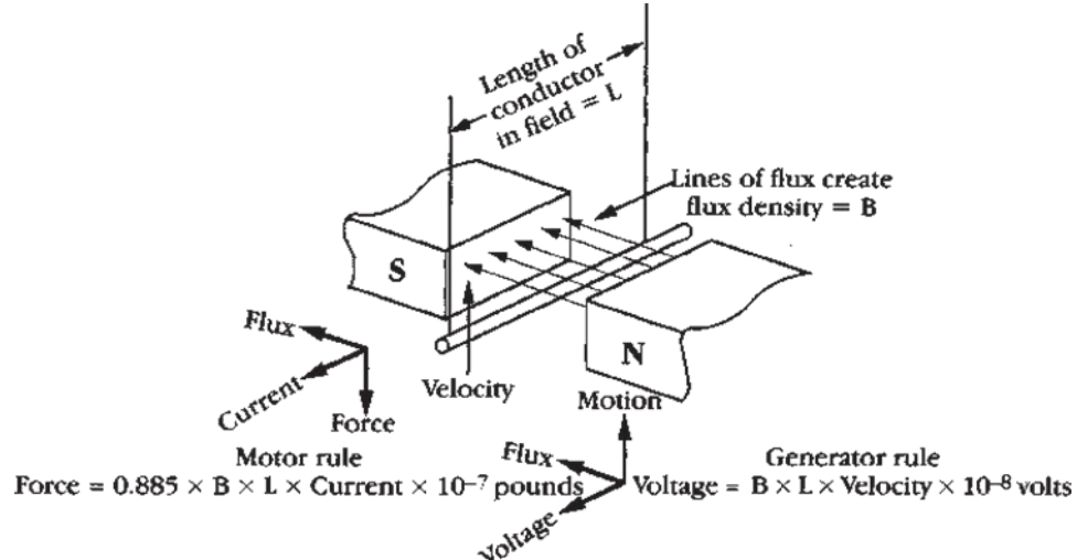
Gambar 6.1 Dasar-dasar motor DC—aturan motor dan generator.
