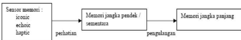
Gambar 2.5 Memori Manusia
