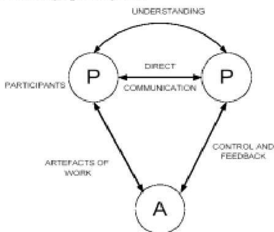
Gambar 10.1 Klasifikasi groupware
