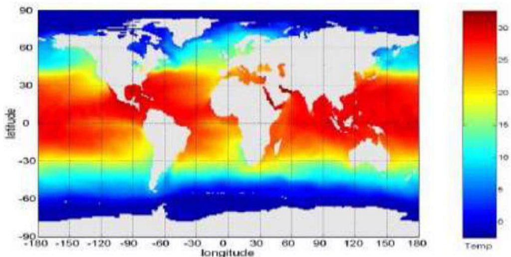
Gambar 11.2 Suhu permukaan laut
