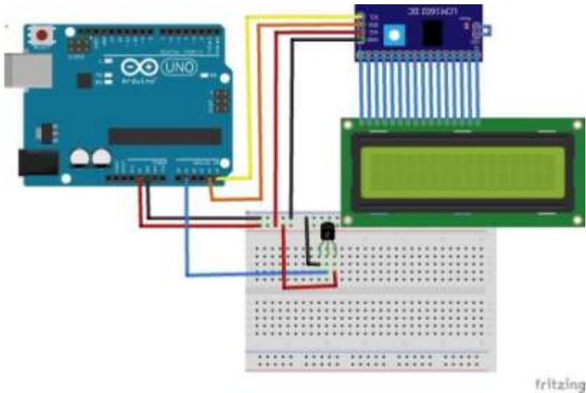
Gambar 16. Skematik LM35 dan LCD I2C
