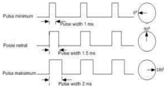
Gambar 26. Posisi sudut motor servo
