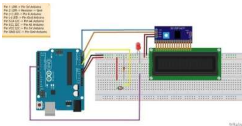
Gambar 19. Skematik LDR dan LCD serta LED
