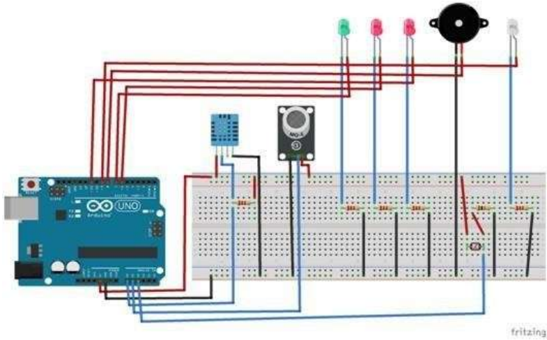
Gambar 37. Skematik Helm Cerdas Proyek
