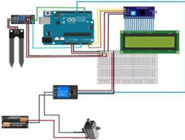
Gambar 40 skematik penyiraman otomatis
