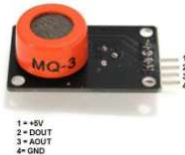
Gambar 30. Pin dalam MQ 3
