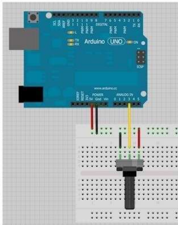
Gambar 17. Skematik arduino dan potensio
