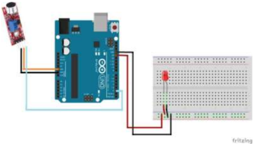
Gambar 35. Skema Pengkabelan arduino led dan sensor suara.
