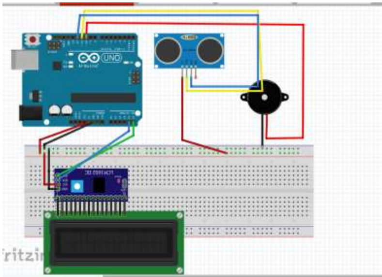
Gambar 24.Skematik HC-SR04,LCDI2C dan Buzzer
