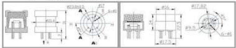
Gambar 30.Komponen MQ7
