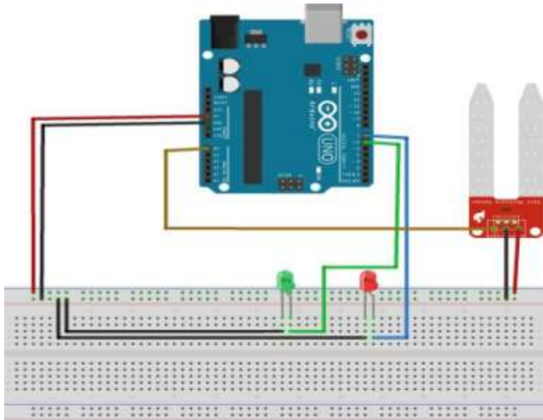
Gambar 24. Skematik Kelembapan tanah dan LED
