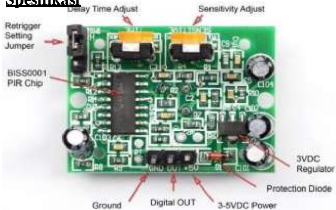
Gambar 21. Bagian-Bagian PIR
