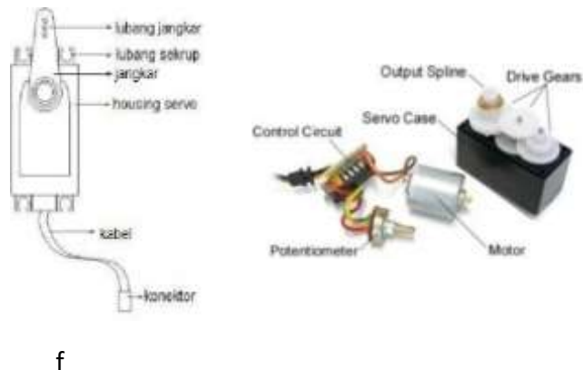
Gambar 26.Komponen Motor Servo
