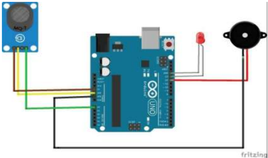
Gambar 32.Skematik MO7 ,Buzzer dan Led
