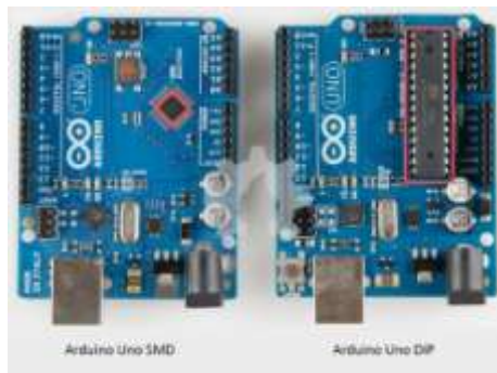
Gambar1.Arduino Uno DIP dan SMD
