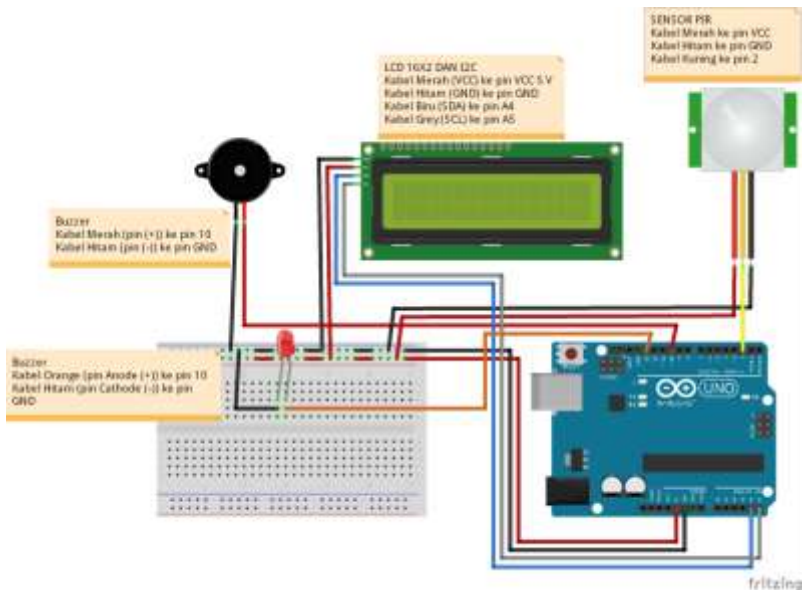
Gambar 22. Skematik PIR, LED, Buzzer dan LCD
