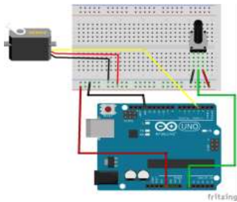
Gambar 28. Skematik Rangkaian
