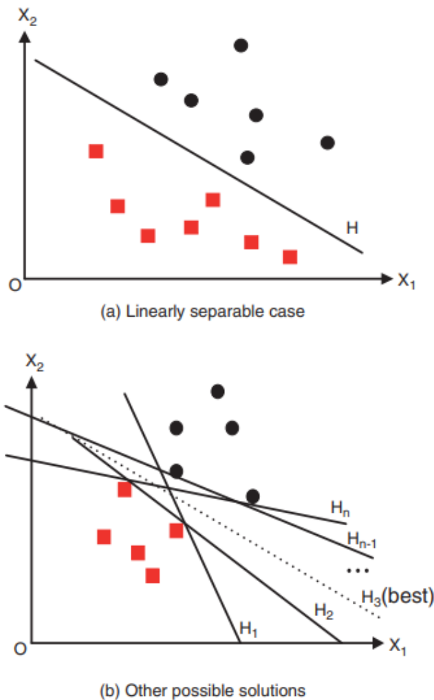
Gambar 4.18 Konsep penggunaan SVM untuk mengklasifikasikan antara dua kelas data sampel.
