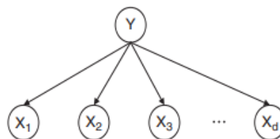
Gambar 2.24 Asumsi independensi bersyarat dari pengklasifikasi Naive Bayesian.
