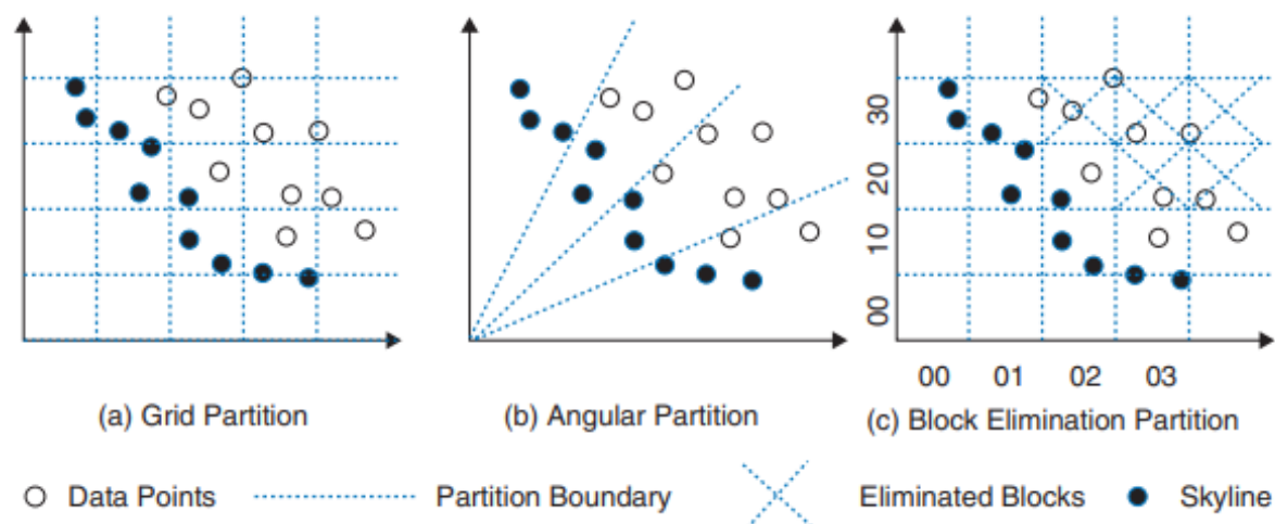
Gambar 2.23 Tiga metode partisi data untuk pemrosesan kueri skyline MapReduce. (Ditetak ulang dengan izin dari F. Zhang, K. Hwang, dkk. 2016 [23]).
