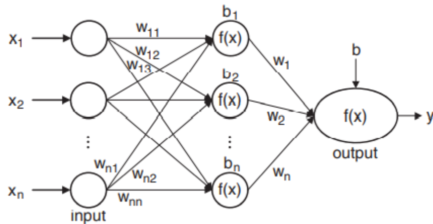
Gambar 6.8 Struktur jaringan syaraf tiruan dua lapis.
