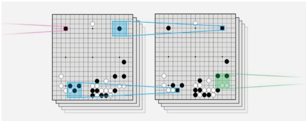
Gambar 8.12 Konstruksi jaringan saraf convolutional di atas papan permainan Go.
