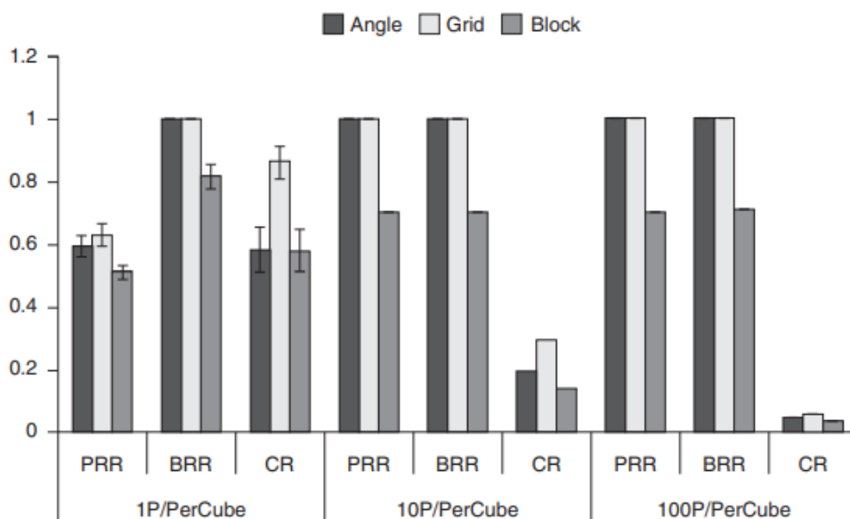
Gambar 2.24 Kinerja relatif dari tiga metode MapReduce untuk kinerja cloud mashup (Dicetak ulang dengan izin dari F. Zhang, K. Hwang, et al., 2016. [23])
