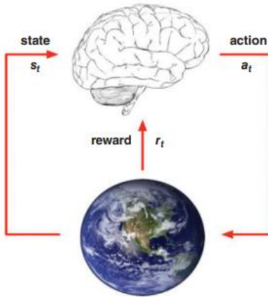
Gambar 8.11 Interaksi agen dan lingkungan dalam Deep learning (dicetak ulang dengan izin dari presentasi David Silver di Konferensi Internasional tentang Machine learning , ICML 2016) [20].
