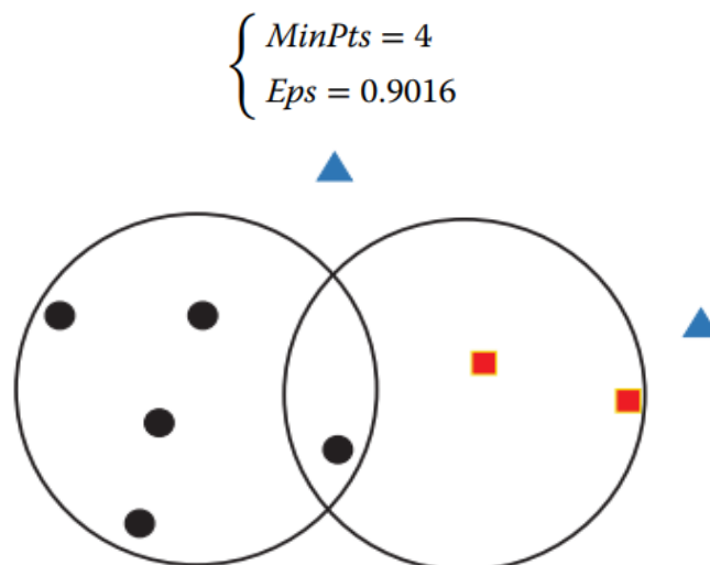
Gambar 5.7 Titik inti, titik perbatasan dan titik kebisingan dalam dua cluster.
