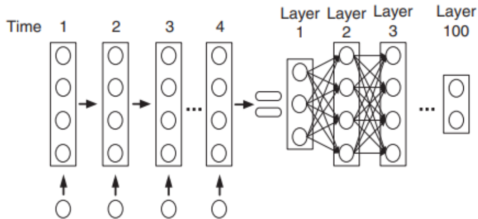
Gambar 6.29 Kontras antara arsitektur RNN dan ANN.
