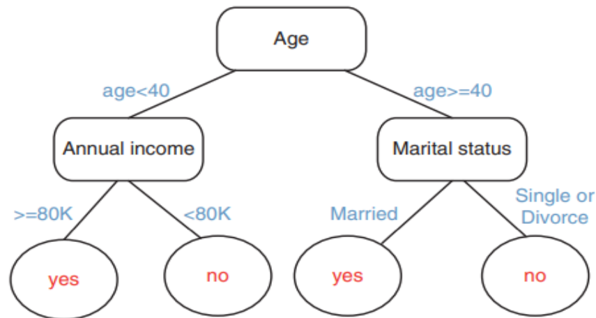
Gambar 4.11 Pohon keputusan untuk menyetujui permohonan pinjaman kepada nasabah bank.
