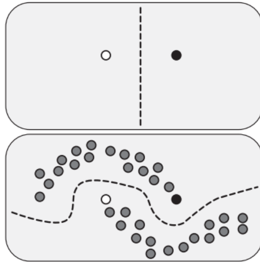
Gambar 5.12 Contoh untuk menggambarkan Machine learning semi-diawasi.
