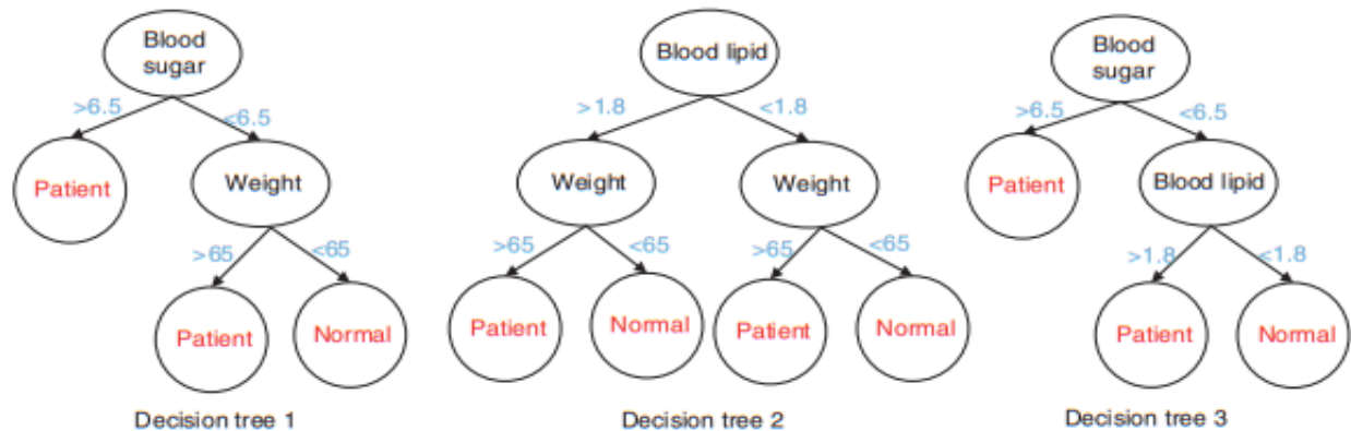
Gambar 4.29 Representasi hutan acak diabetes.
