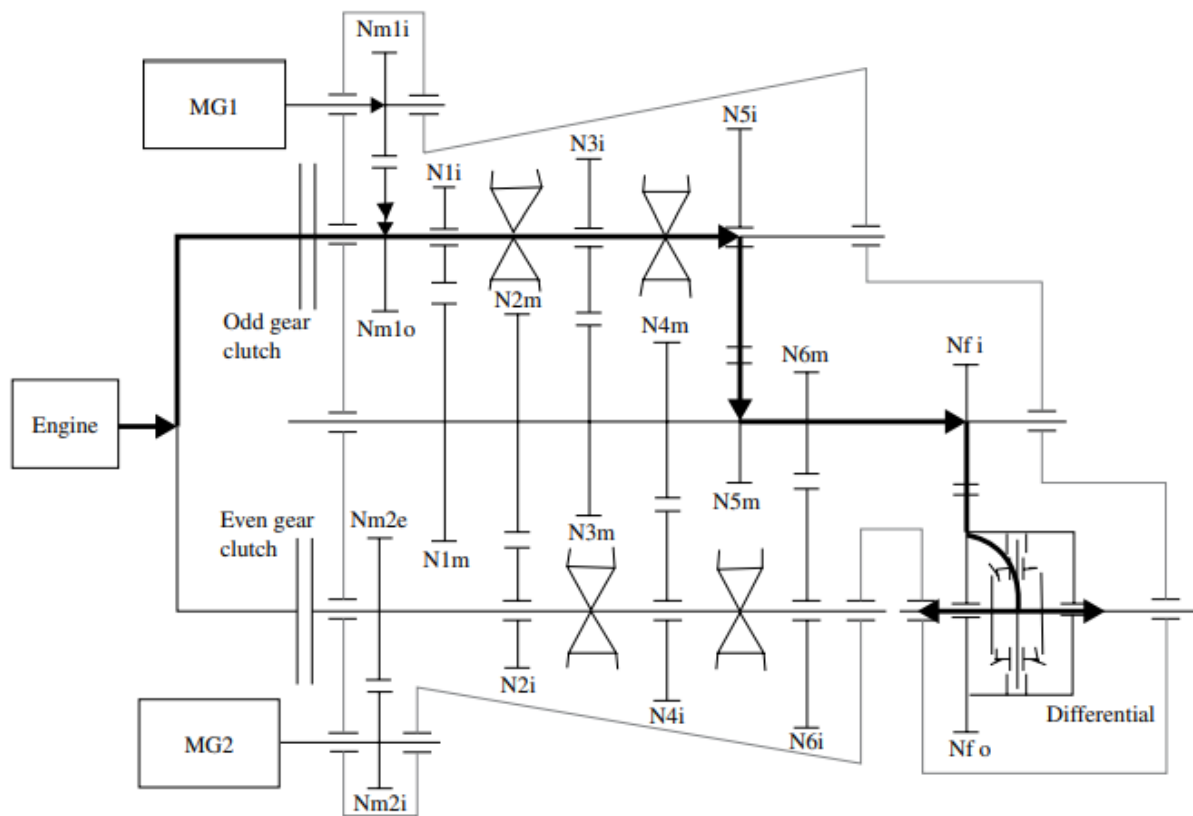
Gambar 4.14 Aliran daya dalam mode kombinasi.
