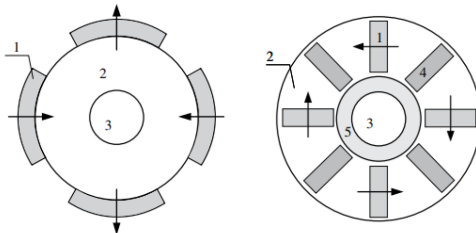
Gambar 10.25 Pemasangan permukaan dan magnet internal: kiri, motor SPM. Benar, motor IPM. 1 - magnet; 2 - inti besi; 3 - poros; 4 - bahan non-magnetik; 5 - bahan non-magnetik;
