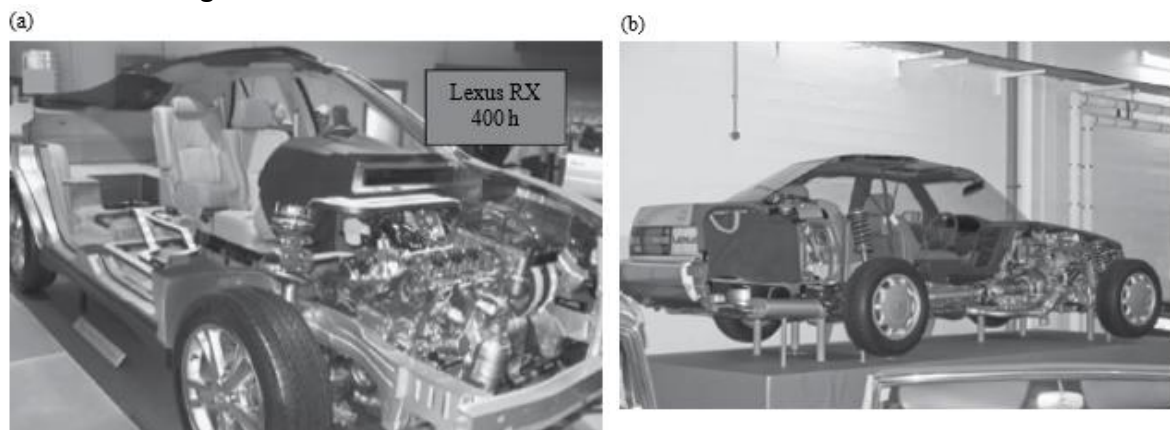
Gambar 2.3 (a) Penampang Lexus RX 400h. (b) Lexus LS 400 cutaway. Atas perkenan Wikimedia,
