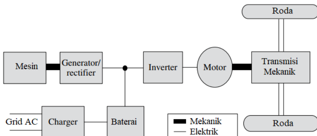
Gambar 5.3 Arsitektur seri PHEV.
