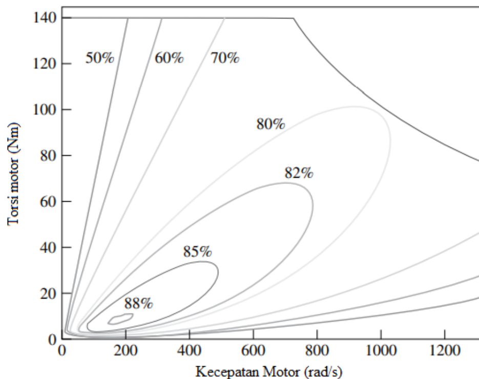
Gambar 3.10 Plot efisiensi motor
