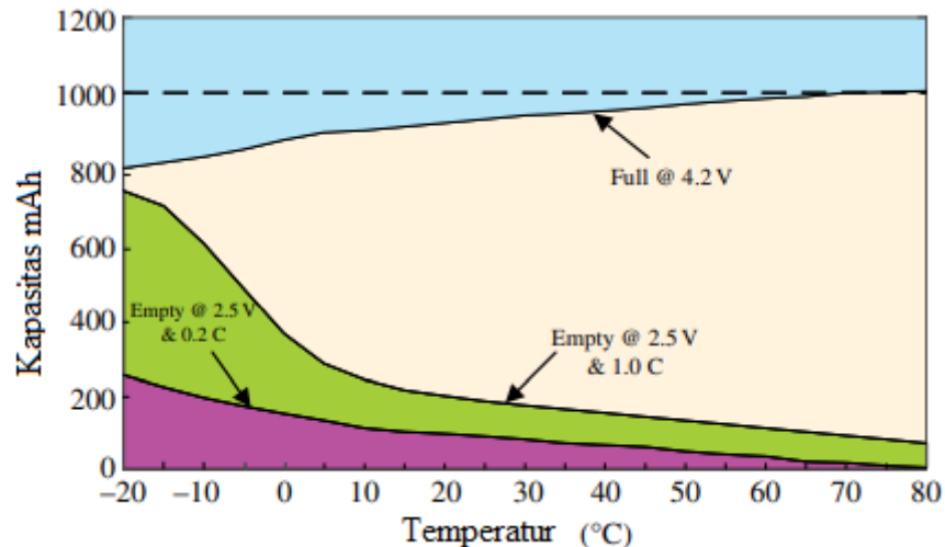
Gambar 11.4 Perubahan kapasitas baterai dengan suhu. Sumber: Dicitak ulang dari mpoweruk.com
