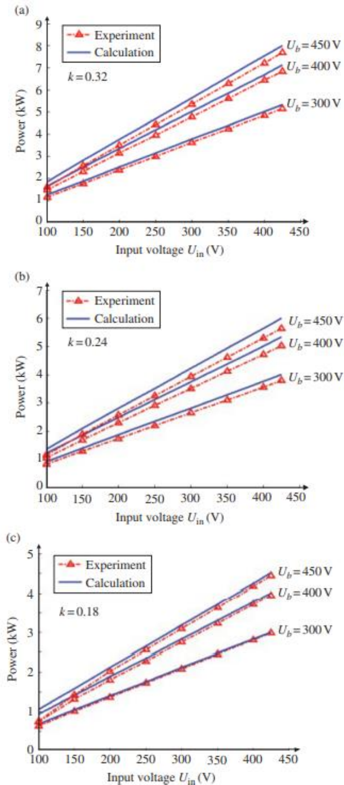
Gambar 16.22 Hasil perhitungan eksperimental dan teoritis tingkat daya untuk sistem pengisi daya nirkabel. (a) k = 0,32 . (b) k = 0,24 . (c) k = 0,18
