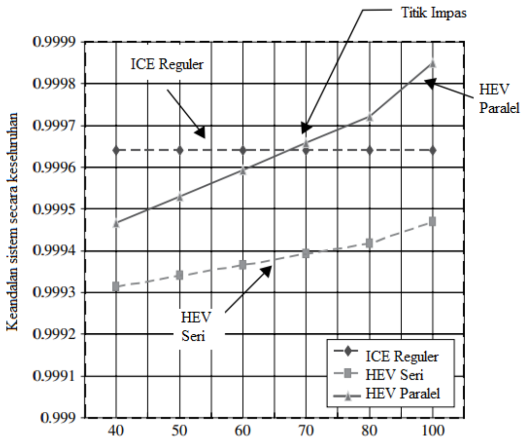
Gambar 8.4 Perbandingan keandalan sistem dan faktor daya yang dirasakan untuk tiga jenis kendaraan yang berbeda. © 2008 IEEE.
