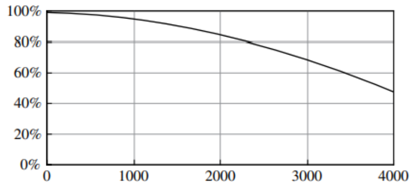
Gambar 5.15 Kapasitas baterai umum versus masa pakai siklus
