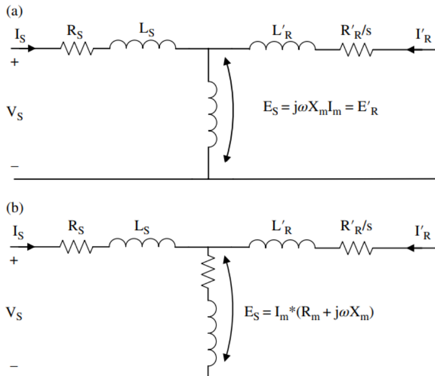
Gambar 10.4 Rangkaian ekivalen yang dimodifikasi dari mesin induksi: (a), mengabaikan rugi-rugi besi; (b), mempertimbangkan kehilangan besi
