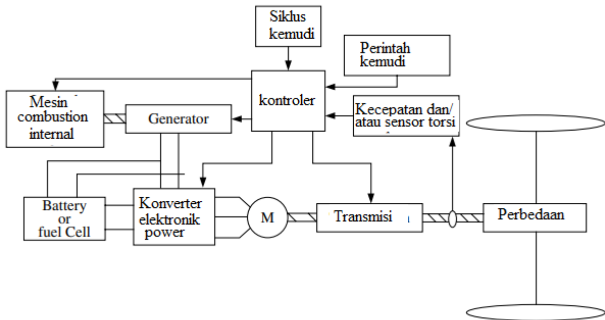
Gambar 14.13 Konfigurasi Seri HEV.
