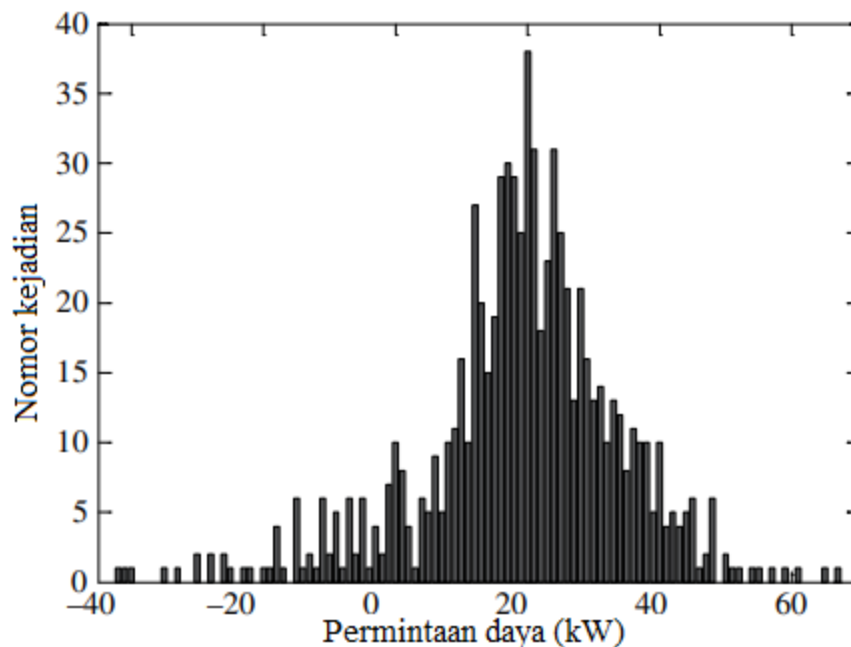
Gambar 5.8 Distribusi permintaan daya dalam mobil penumpang di bawah siklus mengemudi perkotaan UDDS EPA. Sumbu horizontal adalah permintaan daya powertrain, dan sumbu vertikal adalah pembangkitan permintaan daya. Permintaan daya dihitung setiap detik.
