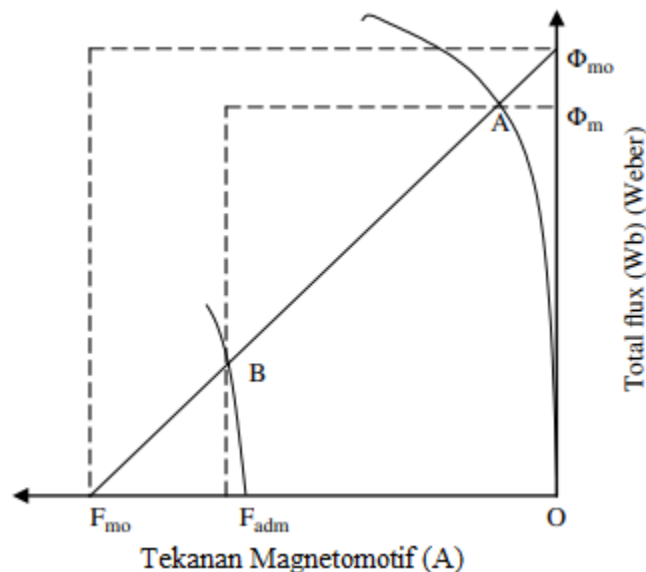
Gambar 10.39 Ilustrasi penggunaan magnet dimana A adalah titik operasi tanpa beban dan B adalah titik arus balik maksimum.
