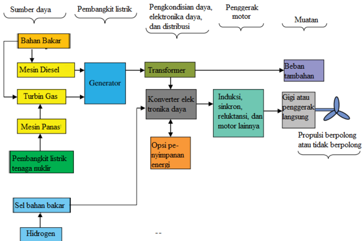
Gambar 6.19 Arsitektur generik sistem kelistrikan kapal. Jalur yang ditunjukkan oleh panah yang memasuki blok tertentu hanya menyiratkan beberapa kemungkinan dan tidak selalu menunjukkan jalur simultan.
