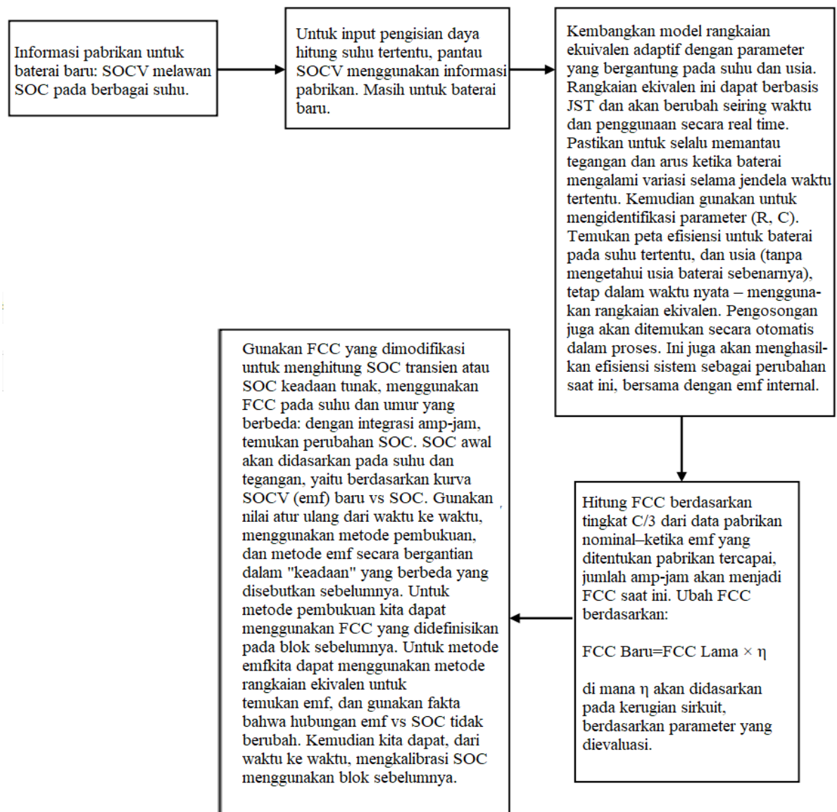
Gambar 11.9 Kemungkinan algoritma untuk perhitungan SOC baterai yang akurat menggunakan adaptasi berbasis model.
