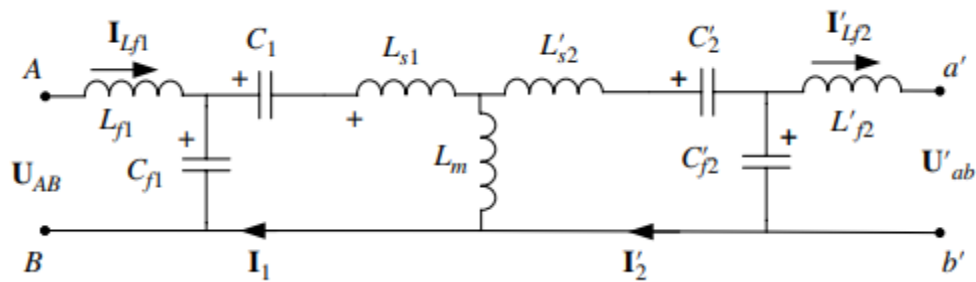
Gambar 16.12 Rangkaian ekivalen mengacu pada sisi utama dari topologi yang diusulkan
