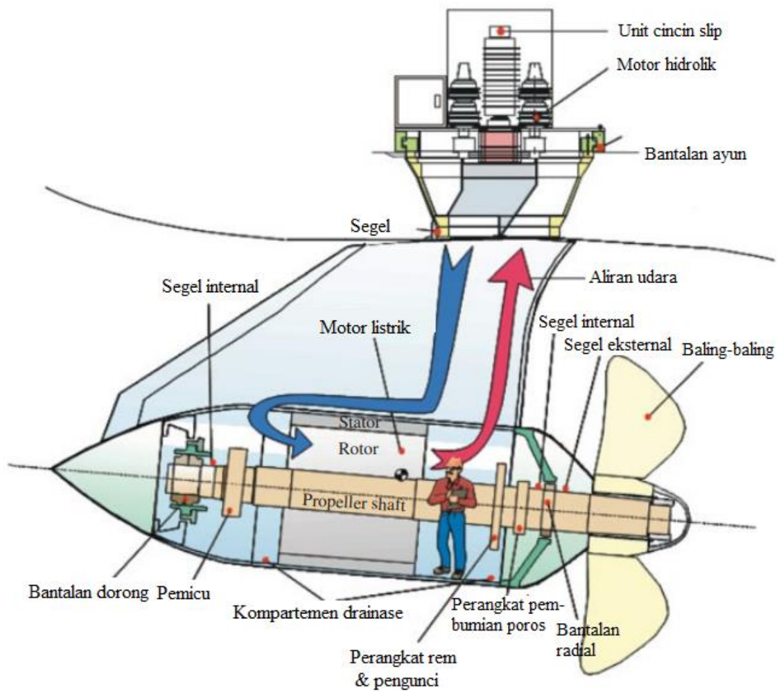
Gambar 6.21 Sistem penggerak pod yang digunakan di atas kapal. Sumber: Courtesy of Rolls-Royce plc.
