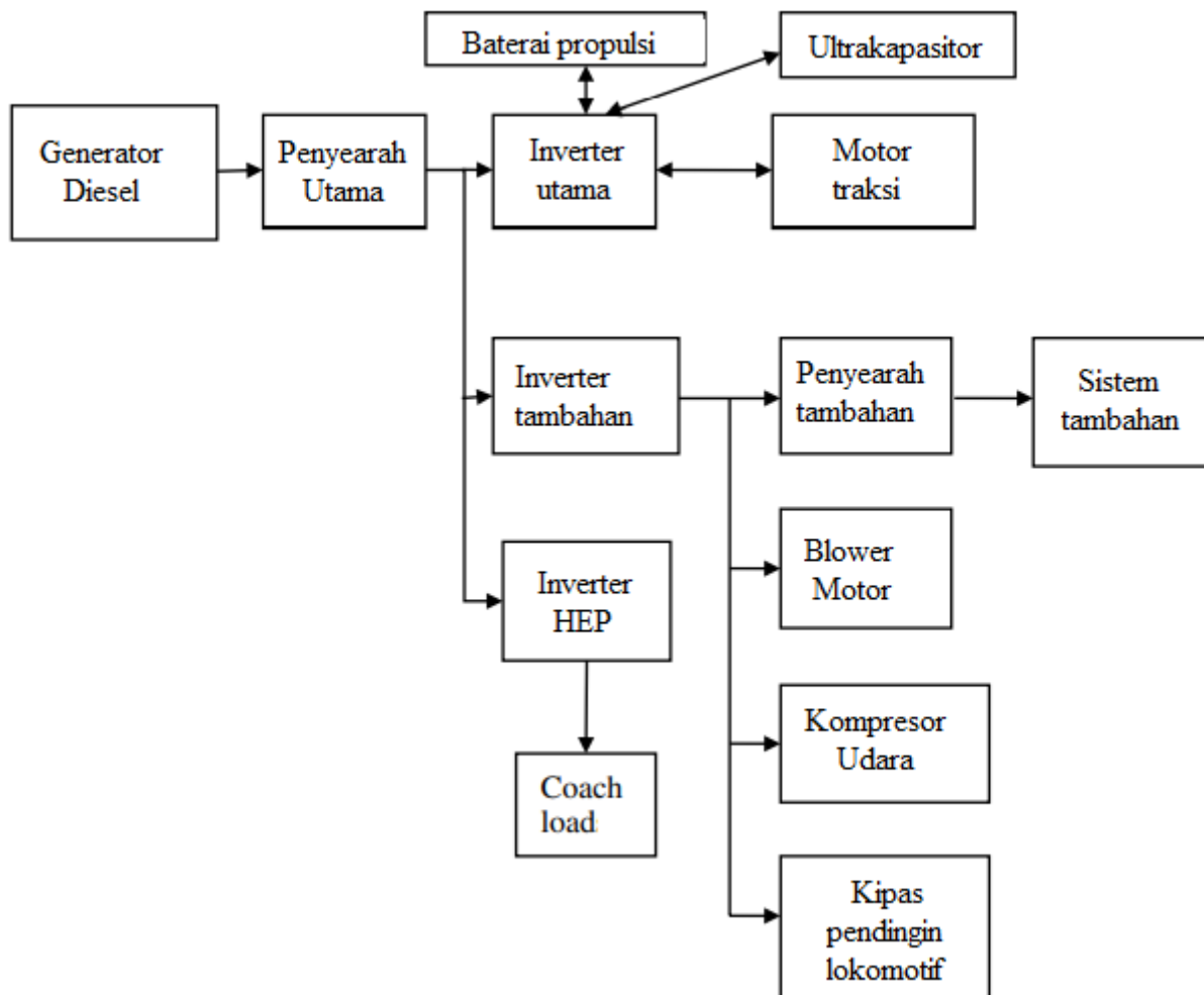
Gambar 6.28 Arsitektur sistem kelistrikan dan propulsi lokomotif diesel-listrik dengan kemampuan pengereman regeneratif.
