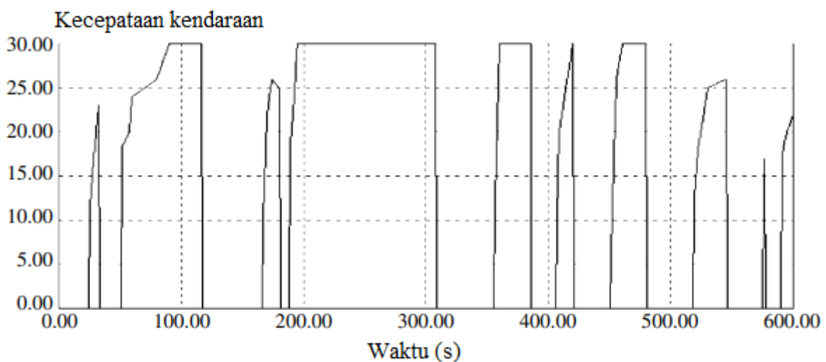
Gambar 14.14 Kecepatan motor ( \times 100 rpm) versus waktu (detik).
