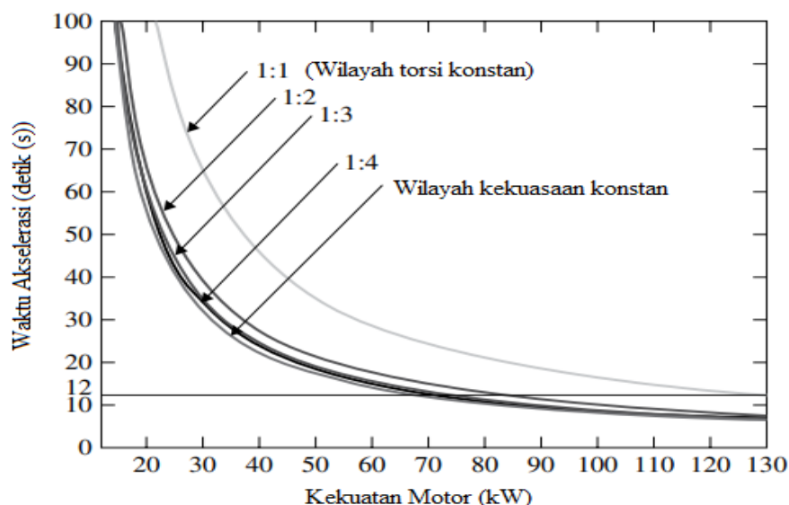
Gambar 3.14 Daya motor sebagai fungsi dari rentang daya konstan.
