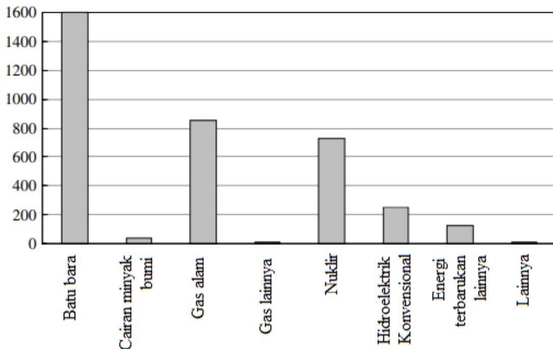
Gambar 5.2 Portofolio pembangkit listrik. Sumber: Administrasi Informasi Energi.
