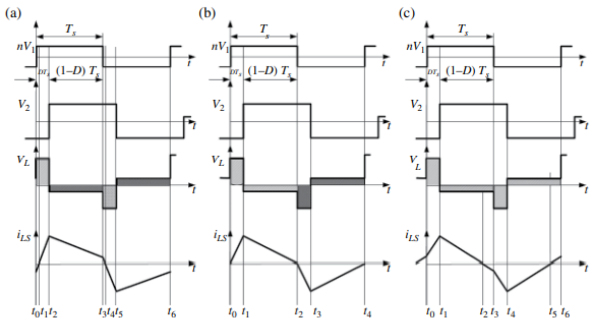
Gambar 9.16 Kurva tegangan dan arus tipikal untuk V_2 > nV_1 : (a) bentuk gelombang untuk i(t_0) < 0 ; (b) bentuk gelombang untuk kondisi batas i(t_0) = 0 ; (c) bentuk gelombang untuk i(t_0) > 0 .
