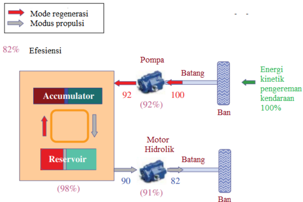
Gambar 6.4 Distribusi Efisiensi Pengereman Regeneratif HHV. Sumber: US EPA 2004.
