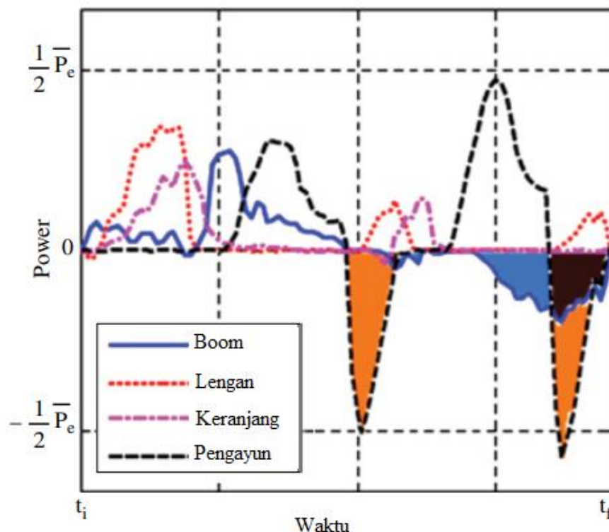
Gambar 6.18 Kebutuhan daya untuk komponen ekskavator. Sumber: Yoo 2009. Dicitak ulang dengan izin dari IEEE.
