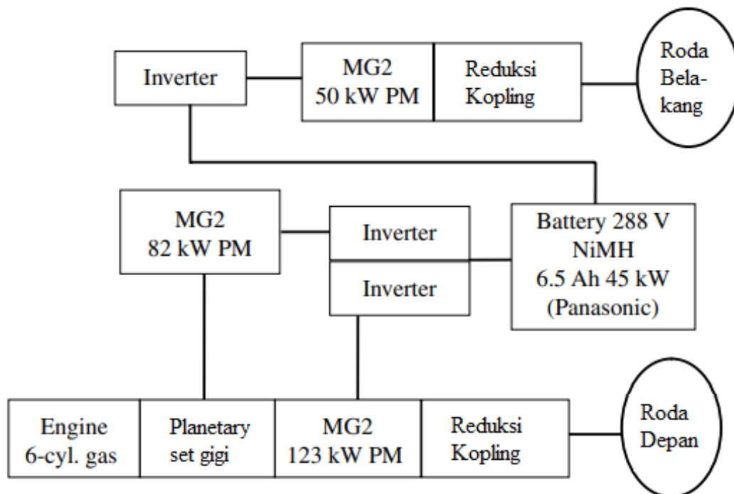
Gambar 4.23 Diagram skema sistem hybrid penggerak empat roda listrik
