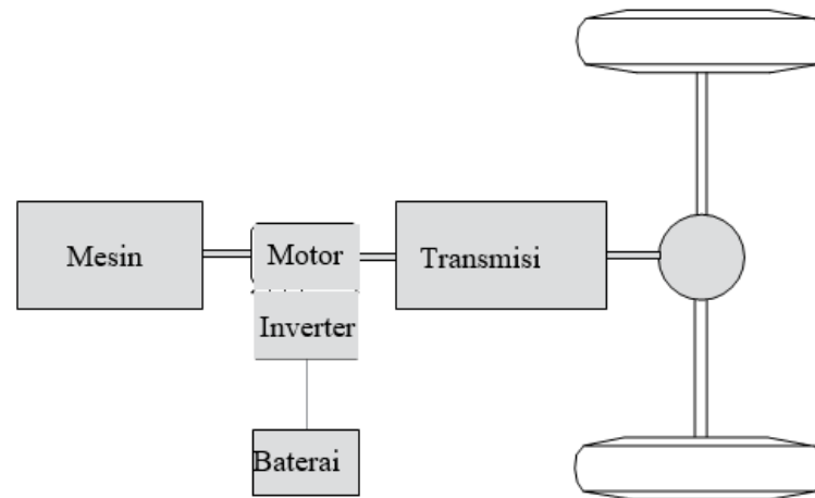
Gambar 1.22 Arsitektur powertrain dari Honda Civic hybrid
