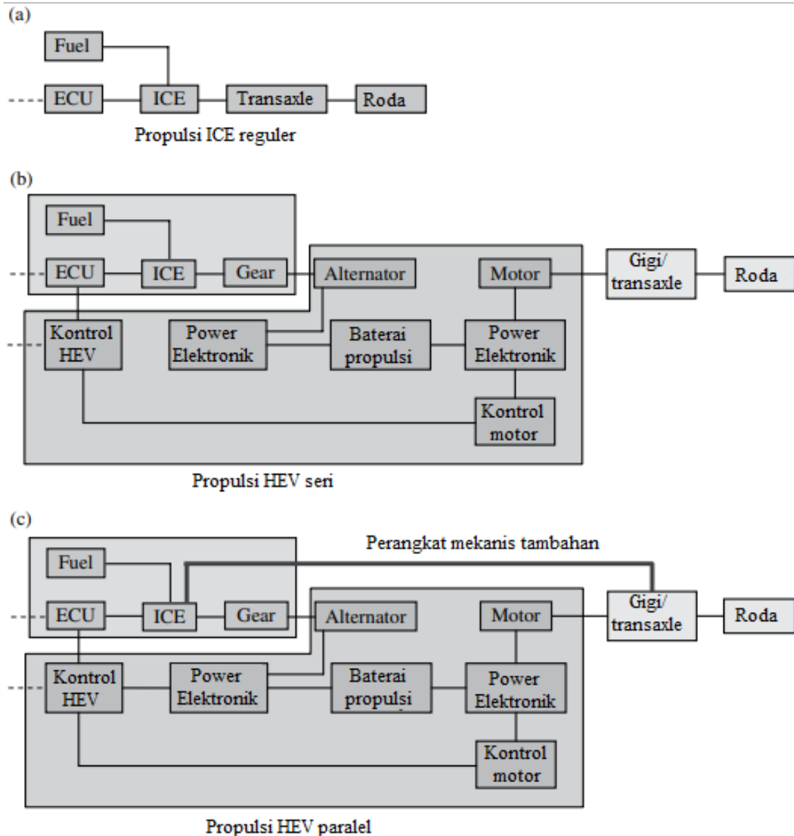
Gambar 8.3 Diagram blok taraf sistem dari (a) ICE reguler, (b) serial HEV, dan (c) arsitektur HEV paralel. © 2008 IEEE.
