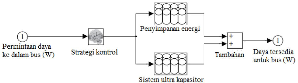
Gambar 14.4 Diagram blok representasi baru dari subsistem baterai yang terdiri dari baterai dan ultrakapasitor. Hubungan input/output dengan sistem lainnya dibiarkan tidak berubah.
