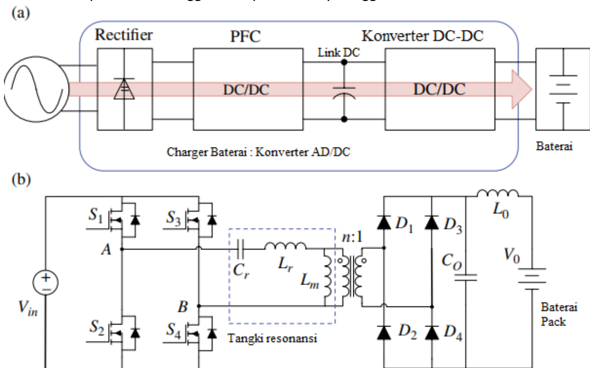
Gambar 13.1 Konverter resonansi full-bridge LLC. (a) Sistem Pengisi Daya EV/PHEV tipikal. (b) Tahap konverter DC–DC LLC untuk Pengisi Daya EV/PHE.
