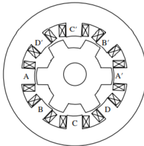
Gambar 10.42 Keengganan sinkron motor.
