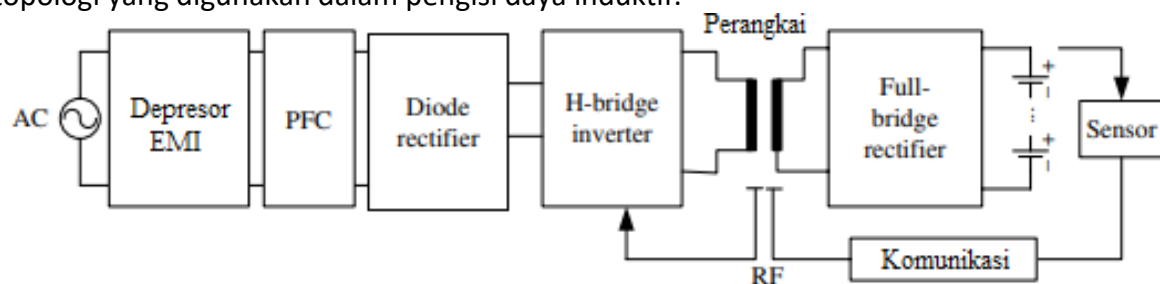
Gambar 9.34 Pengisi daya induktif terisolasi.
