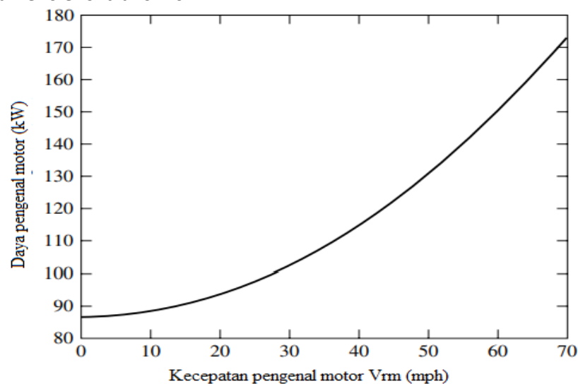
Gambar 3.13 Daya pengenal motor sebagai fungsi kecepatan pengenal motor selama akselerasi.
