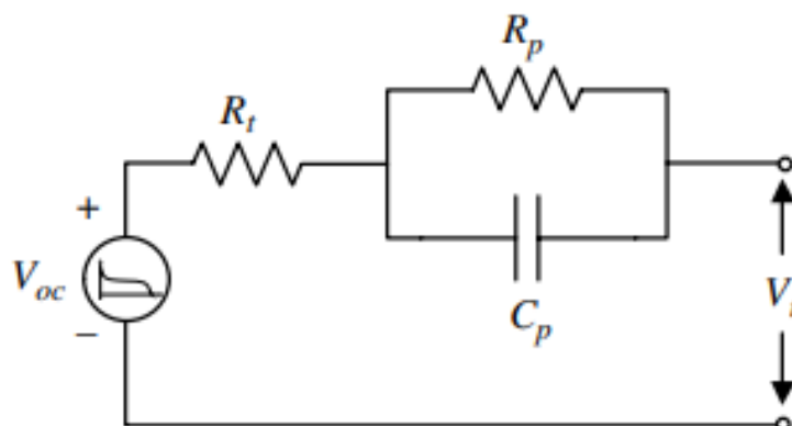
Gambar 12.4 Model rangkaian ekuivalen orde pertama dari baterai.
