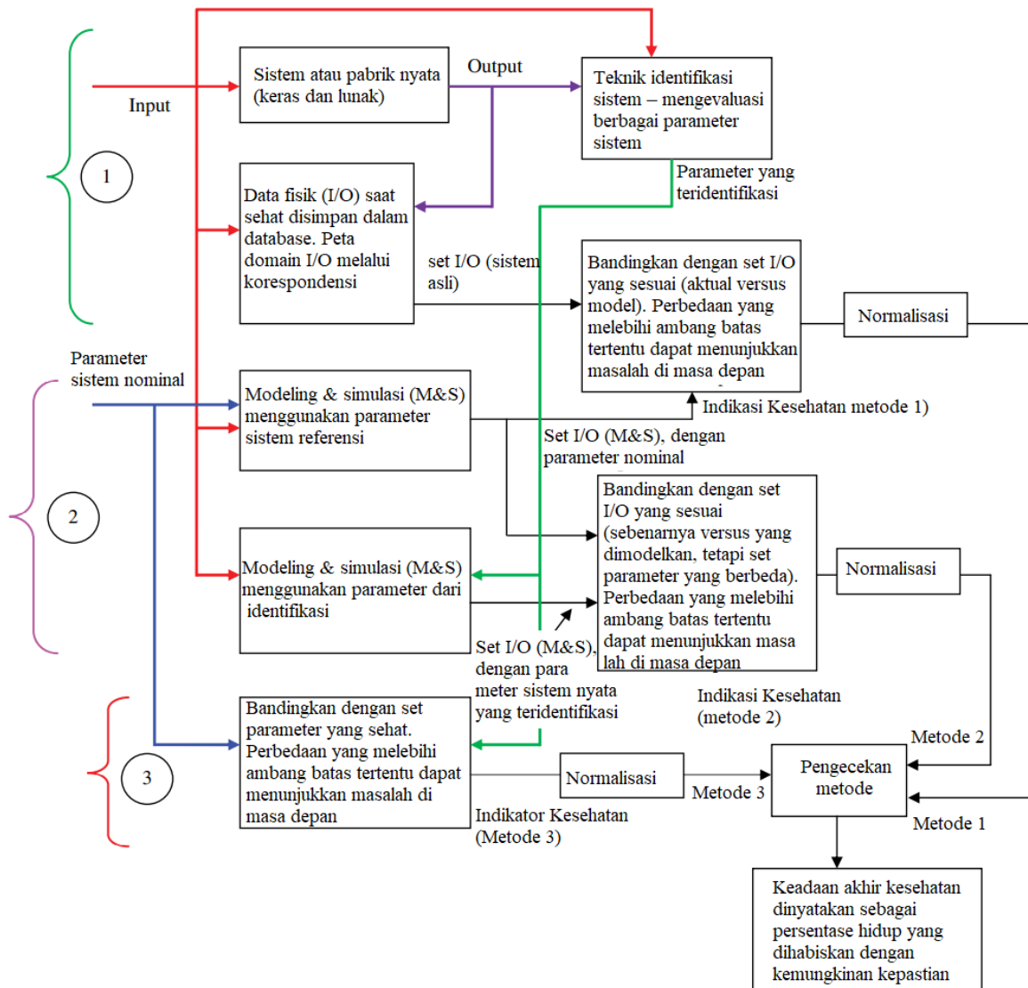
Gambar 8.2 Metodologi umum yang menjelaskan kuantifikasi status kesehatan (konsep dasar dirangkum dalam Tabel 8.1).
