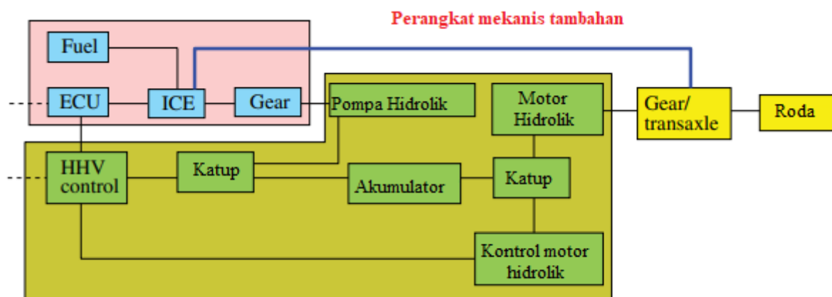
Gambar 6.2 Diagram level sistem HHV. Sumber: Masrur 2008. Dicitak ulang dengan izin dari IEEE.
