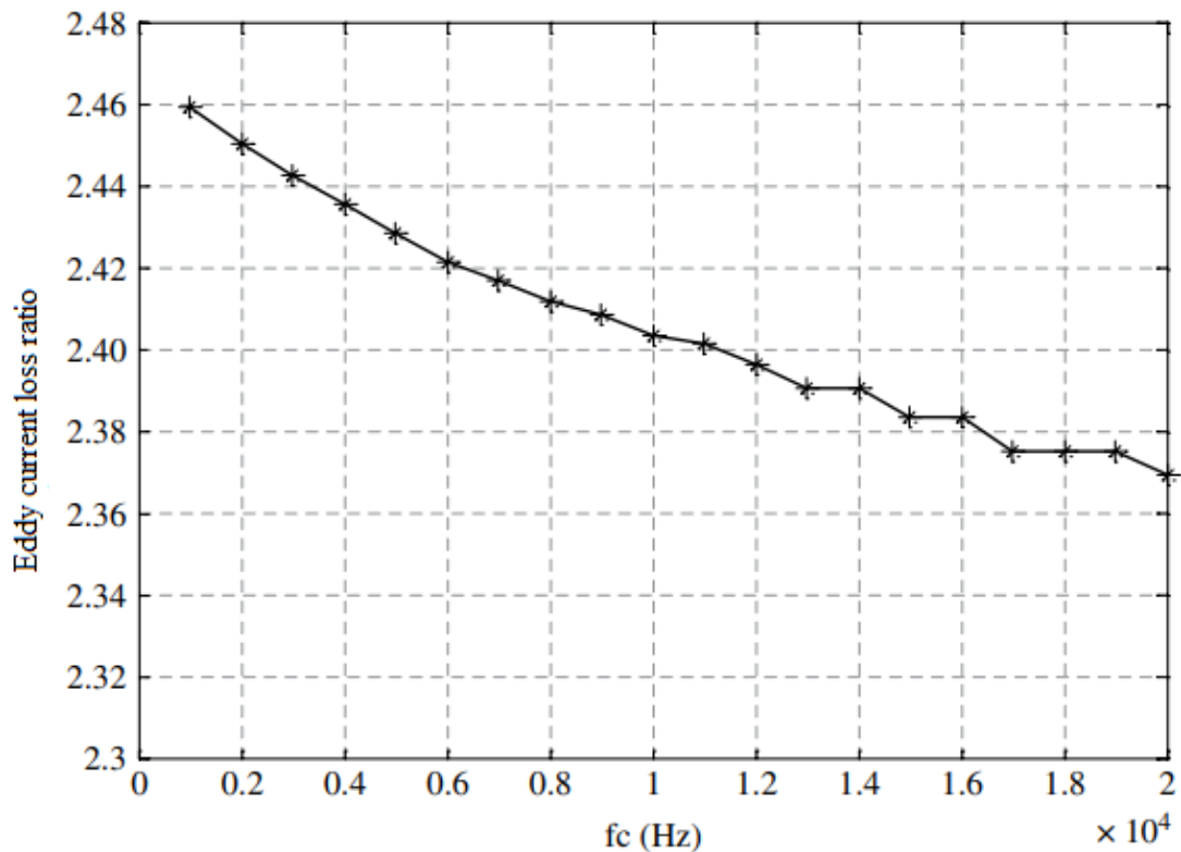
Gambar 10.11 Faktor rugi arus Eddy versus frekuensi switching pada m_a = 0,9
