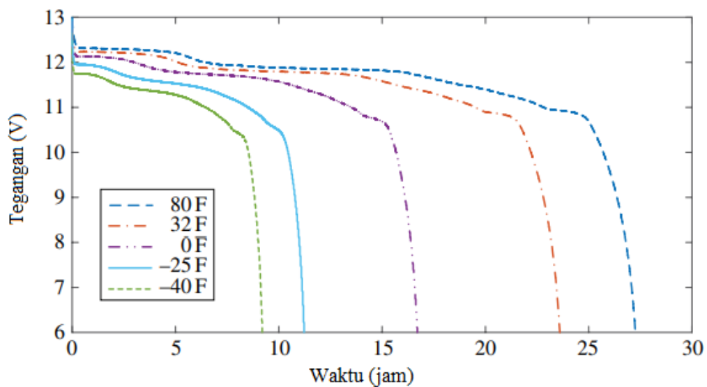
Gambar 11.6 Karakteristik Pengosongan Baterai - Tegangan Terminal pada Laju Pengosongan 5 A (Lembar Data Baterai Keluar).
