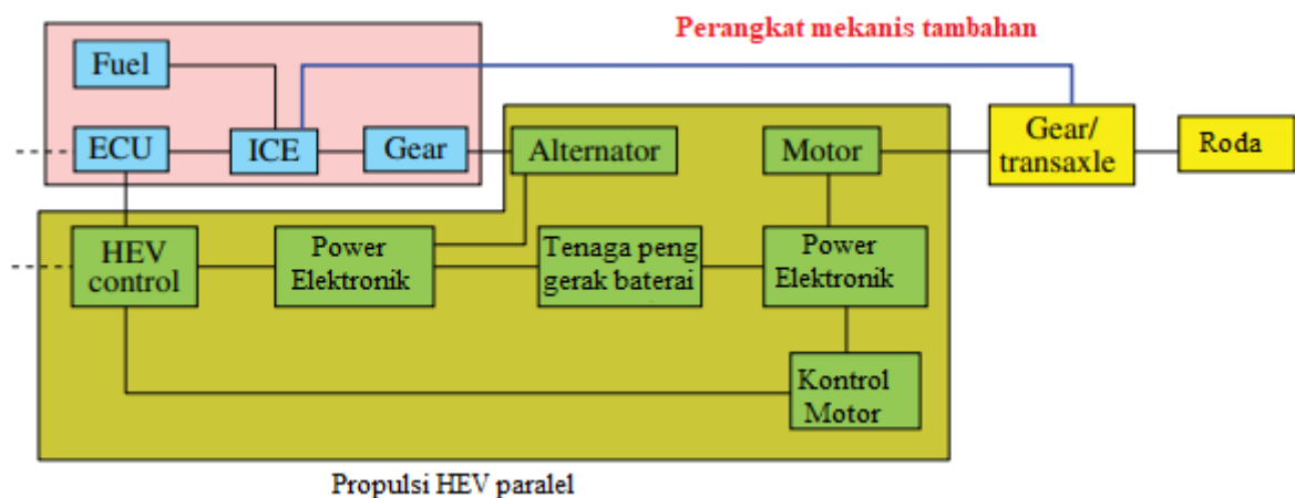
Gambar 6.1 Diagram Level Sistem HEV (ECU, Unit Kontrol Engine, ICE, Mesin Pembakaran) Sumber: Mazur 2008. Dicitak ulang dengan izin dari IEEE.
