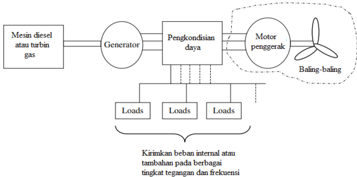
Gambar 6.20 Arsitektur sistem kapal listrik hibrida.
