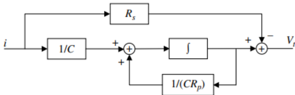
Gambar 11.20 Representasi simulasi rangkaian ekivalen pada Gambar 11.19.
