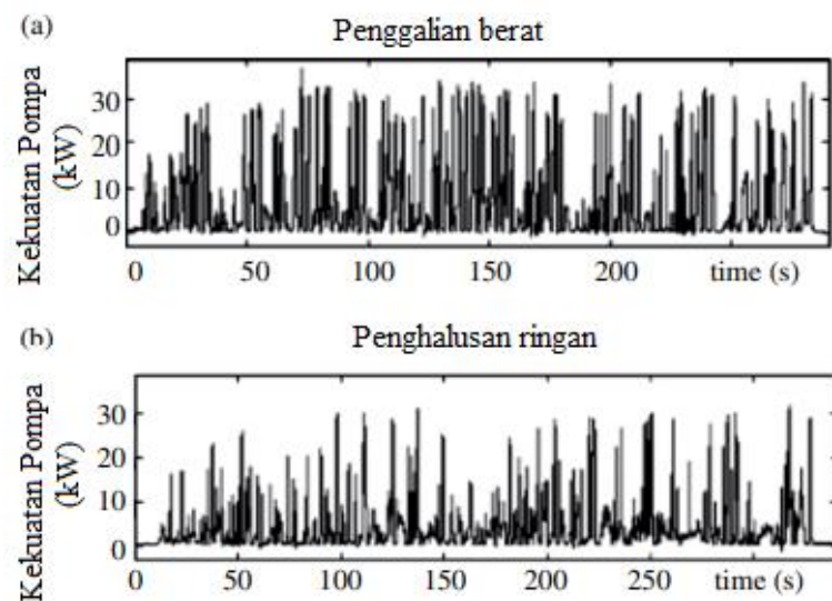
Gambar 6.16 Permintaan beban ekskavator hibrid. Sumber Wang 2008. Dicitak ulang dengan izin IEEE.
