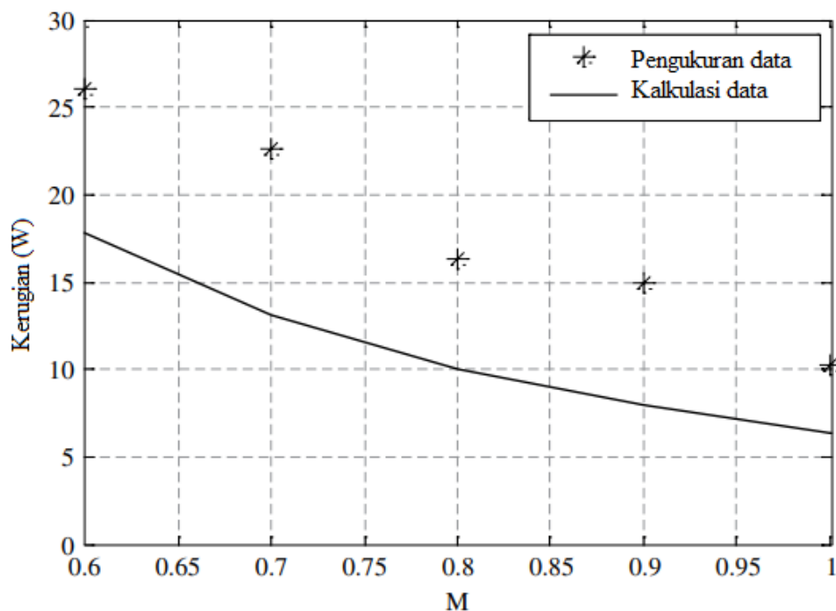
Gambar 10.12 Pengaruh rasio modulasi amplitudo pada kerugian inti motor induksi PWM untuk motor induksi 2 hp.
