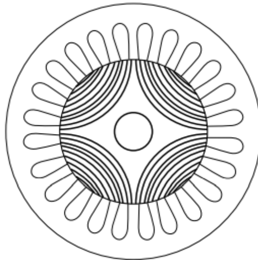
Gambar 10.42 Keengganan sinkron motor.
