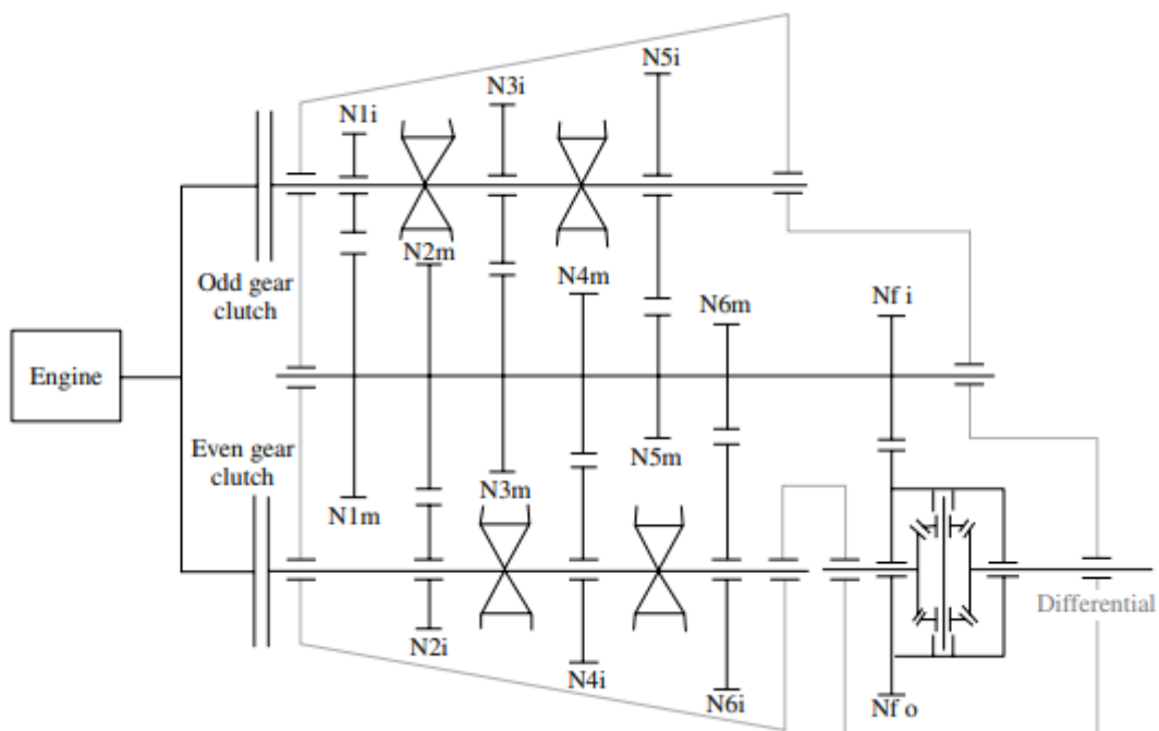
Gambar 4.11 Transmisi kopling ganda. Perhatikan bahwa gigi mundur dihilangkan pada gambar.
