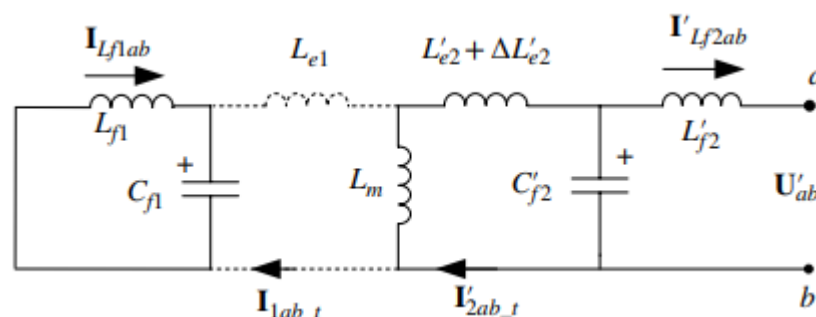
Gambar 16.14 Rangkaian ekuivalen mengacu pada sisi primer.
