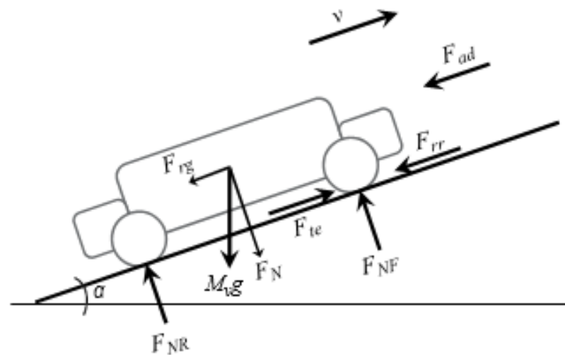
Gambar 3.1 Model Kendaraan
