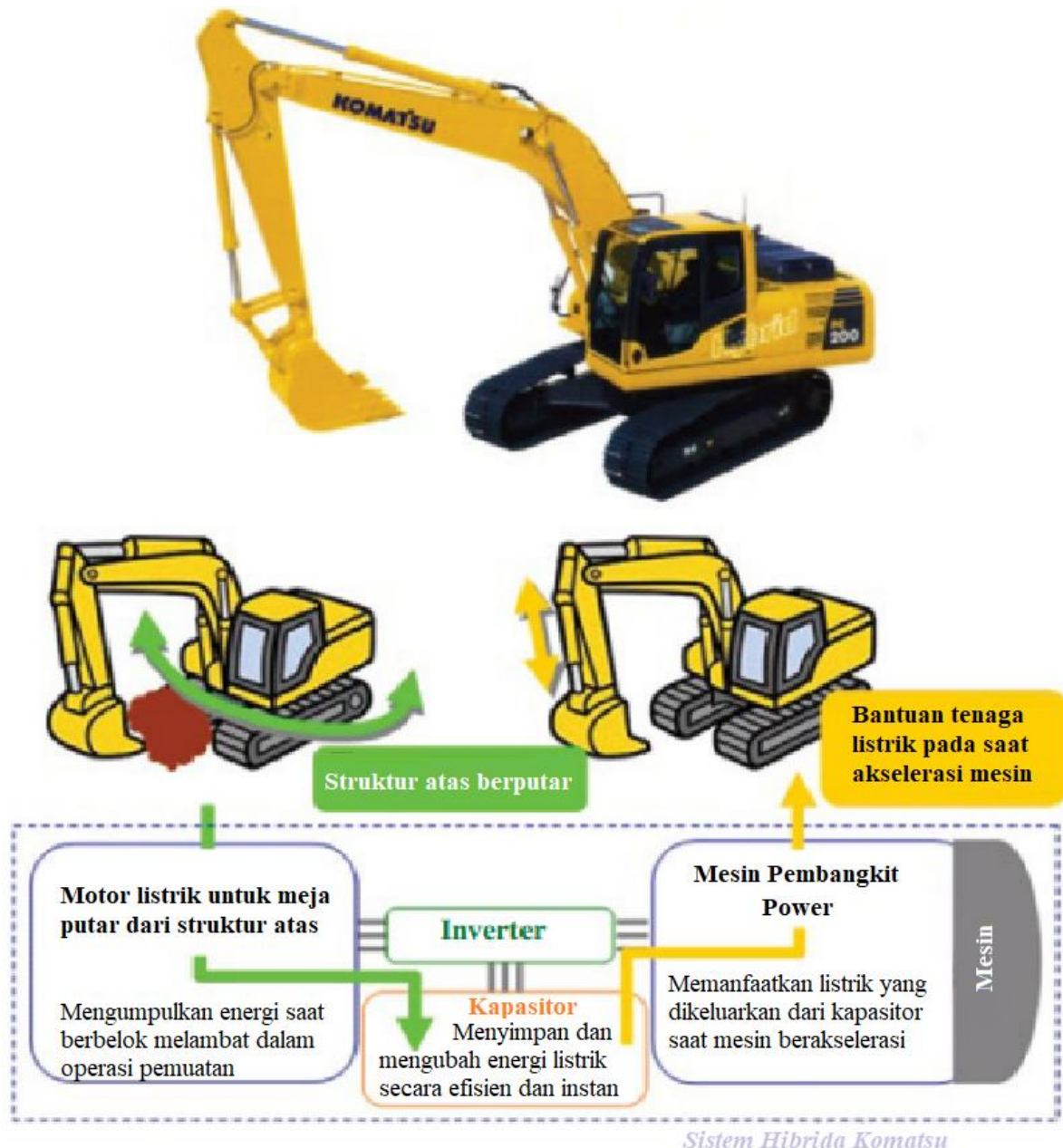
Gambar 6.15 Sistem ekskavator hibrida Komatsu. Sumber: Komatsu
