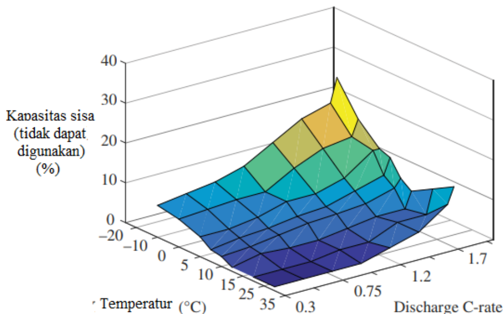
Gambar 11.7 Pengurangan kapasitas baterai pada suhu dan laju pengosongan yang berbeda
