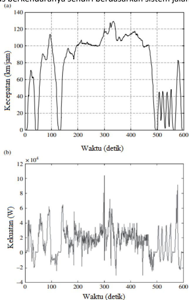
Gambar 3.4 (a) drive cycle US06 dan (b) kendaraan membutuhkan energi listrik pada drive cycle US06.
