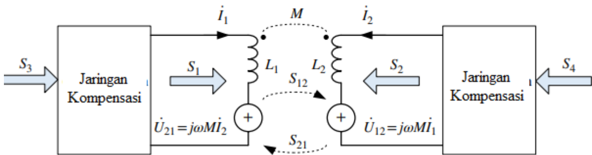
Gambar 16.2 Sistem transfer daya nirkabel dua kumparan umum.
