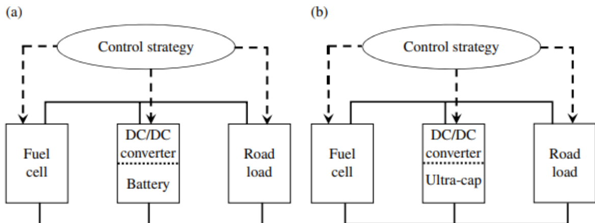
Gambar 3.7 Konfigurasi powertrain hybrid sel bahan bakar.
