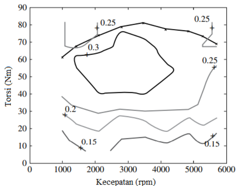
Gambar 14.2 Peta efisiensi mesin penyalan percikan Geo 1,0 l (43 kW).
