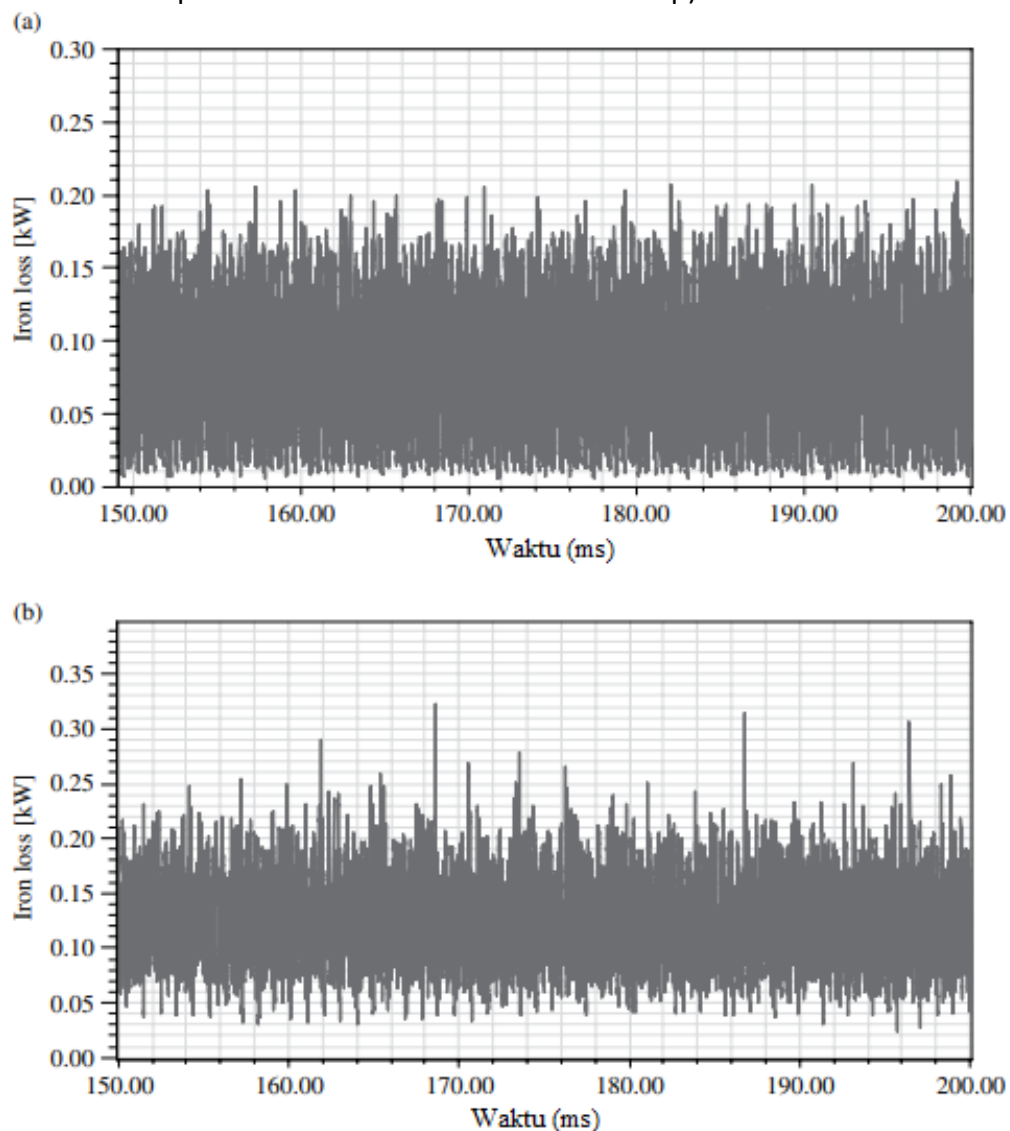
Gambar 10.16 Kehilangan PWM dari simulasi: (a) tanpa beban, (b) dengan beban.
