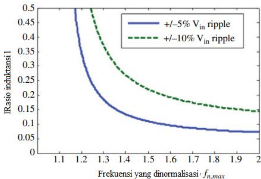
Gambar 13.6 Hubungan antara rasio induktansi dan frekuensi maksimum yang dinormalisasi dalam kondisi tanpa beban.
