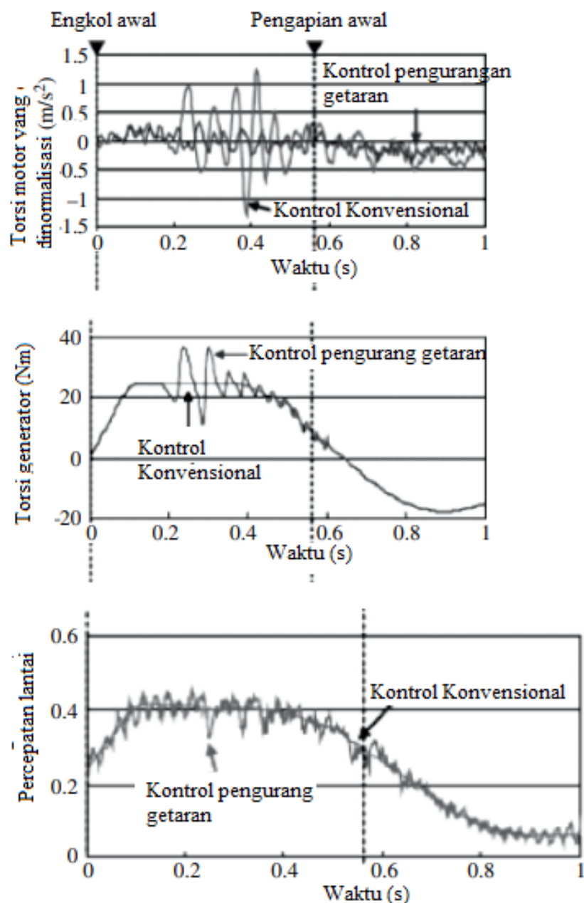
Gambar 8.10 Perbandingan kualitatif pengurangan getaran dengan intervensi kontrol. Panah menunjukkan garis yang menunjukkan kontrol konvensional dan garis yang menunjukkan kontrol reduksi getaran yang diusulkan dalam Gambar. Review R&D Toyota CRDL, vol.40, No.2, hal. 42
