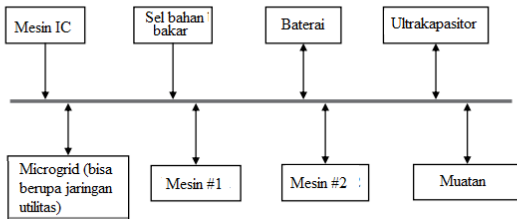
Gambar 7.2 Arsitektur sistem tenaga hibrida biasa.
