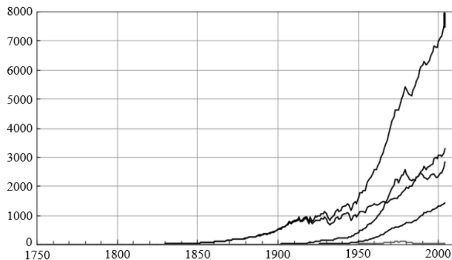
Gambar 1.5 Emisi karbon fosil global mulai 1800 sampai 2004. Di titik ujung kanan, dari atas ke bawah: total CO 2 , minyak, batubara, produksi semen, dan lainnya. Sumber: ONRL.
