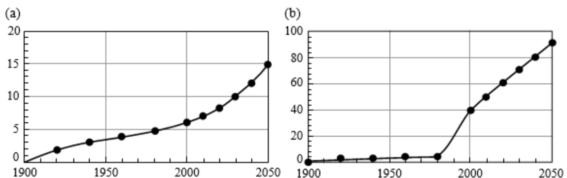
Gambar 1.2 Perubahan populasi dunia dan volume penjualan dua tahun. (a) Populasi dunia dalam miliaran. (b) Jutaan mobil penumpang terjual setiap tahun.
