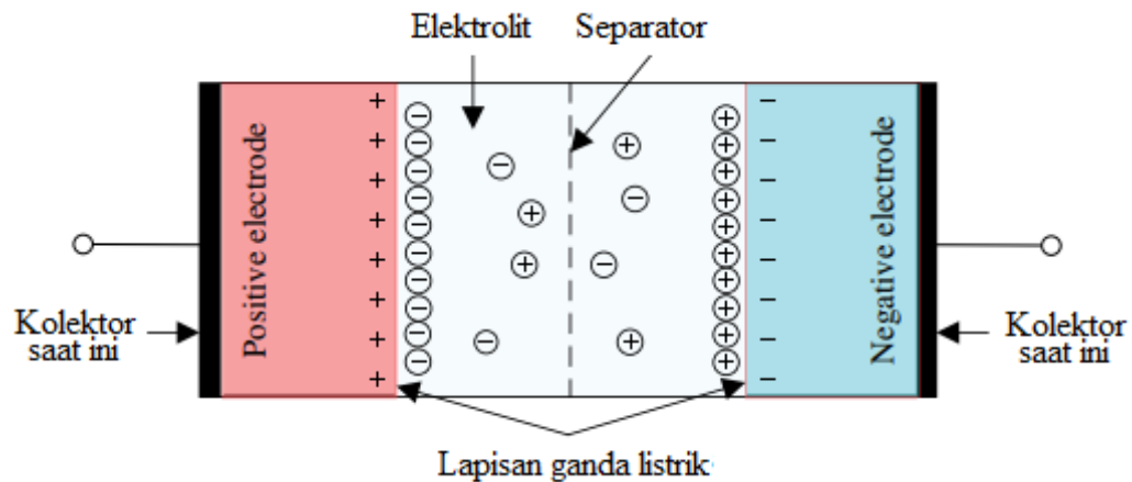
Gambar 11.18 Struktur ultrakapasitor
