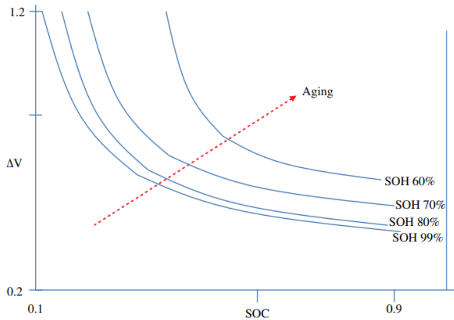
Gambar 11.12 Perubahan tegangan baterai dengan penuaan, SOC dan SOH
