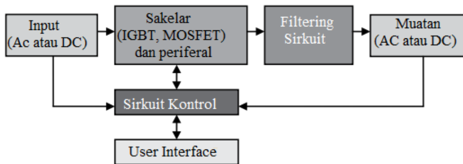
Gambar 9.3 Diagram rangkaian konverter daya
