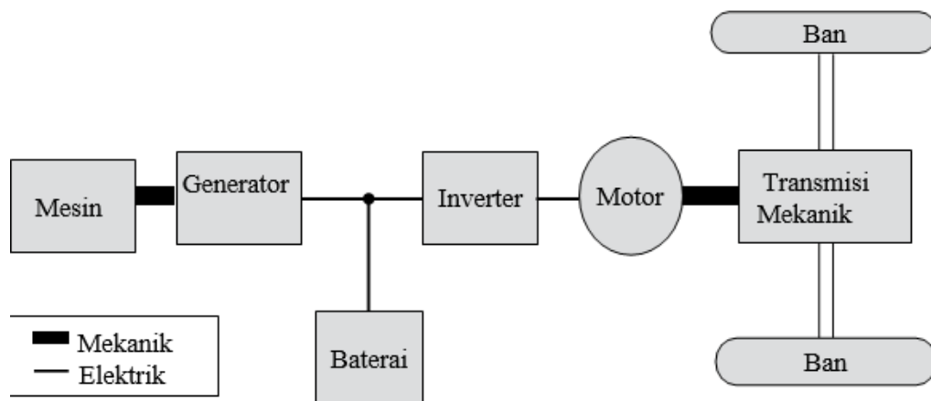
Gambar 1.11 Kerangka seri HEV
