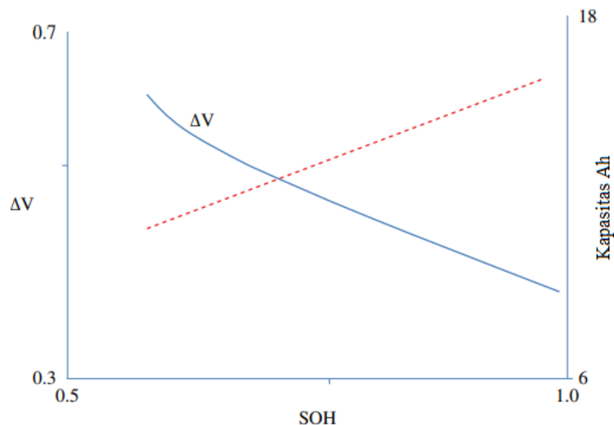
Gambar 11.13 Perubahan tegangan baterai dan kapasitas ampere-hour untuk SOH.
