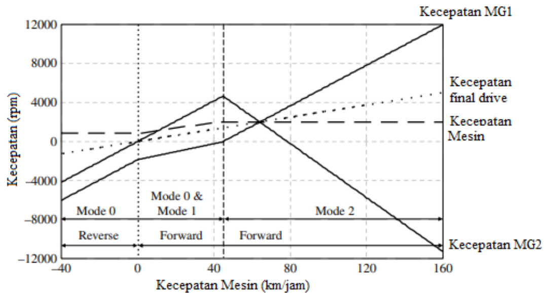
Gambar 4.9 Hubungan kecepatan transmisi dua mode
