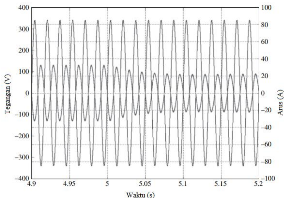
Gambar 5.29 Tegangan input dan arus input 180° keluar fase selama pemakaian.
