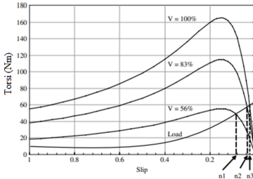
Gambar 10.7 Menyesuaikan kecepatan motor induksi menggunakan catu daya frekuensi variabel. Dalam contoh ini, kecepatan nominalnya adalah 6000 rpm dan kecepatan maksimumnya adalah 12000 rpm. Rentang penyesuaian kecepatan X=2 .
