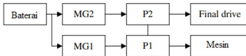
Gambar 4.5 Aliran arus selama startup dan pencadangan
