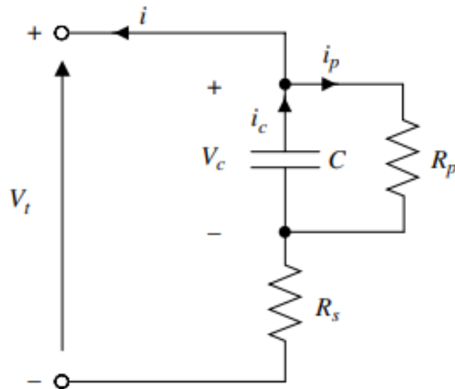
Gambar 11.19 Rangkaian ekivalen ultrakapasitor.
