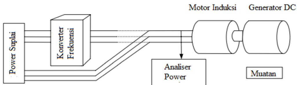
Gambar 10.14 Meja percobaan.
