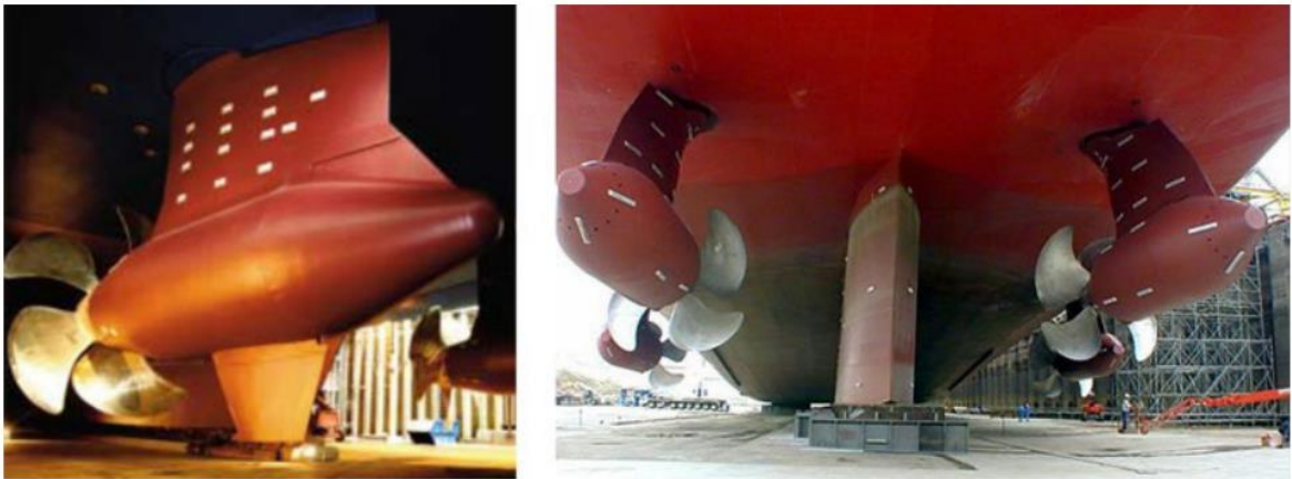
Gambar 6.22 Tampilan sistem propulsi pod yang sebenarnya di kapal: Kiri, Azipod® ABB Oy. Itu benar, Pod Putri Duyung Rolls-Royce. Sumber: Courtesy of Rolls-Royce plc.
