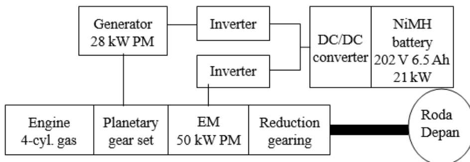
Gambar 1.21 Komposisi powertrain Toyota Prius (EM, mesin listrik; PM magnet permanen).
