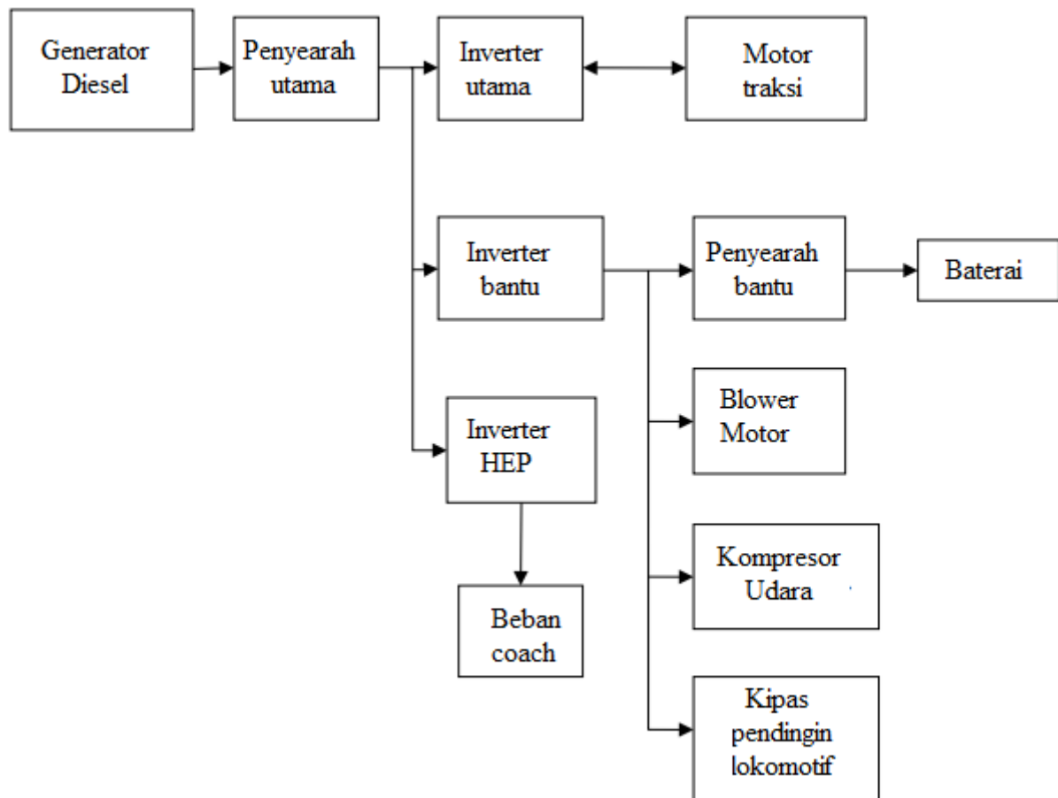
Gambar 6.25 Arsitektur kelistrikan lokomotif diesel dan sistem propulsi.
