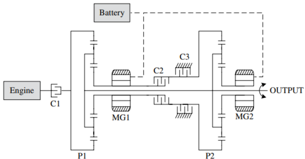
Gambar 4.4 Transmisi hibrid dua mode GM
