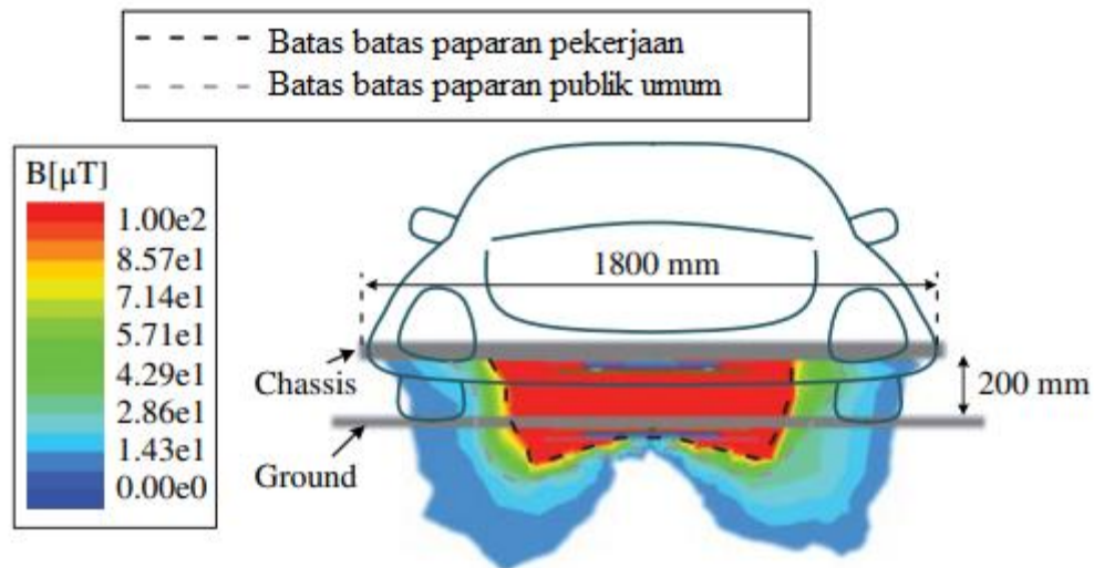
Gambar 16.10 Batas batas pemaparan untuk sistem WPT 8 kW.
