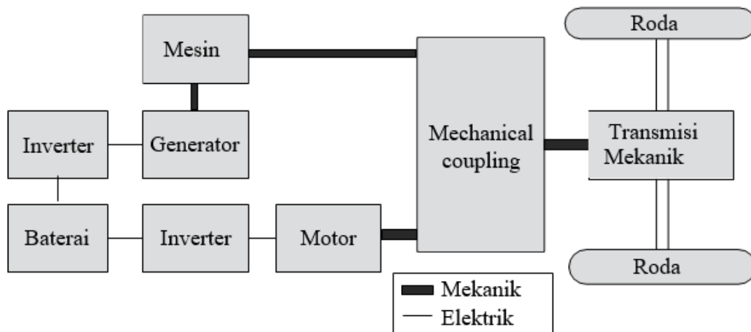
Gambar 1.14 Arsitektur seri paralel HEV
