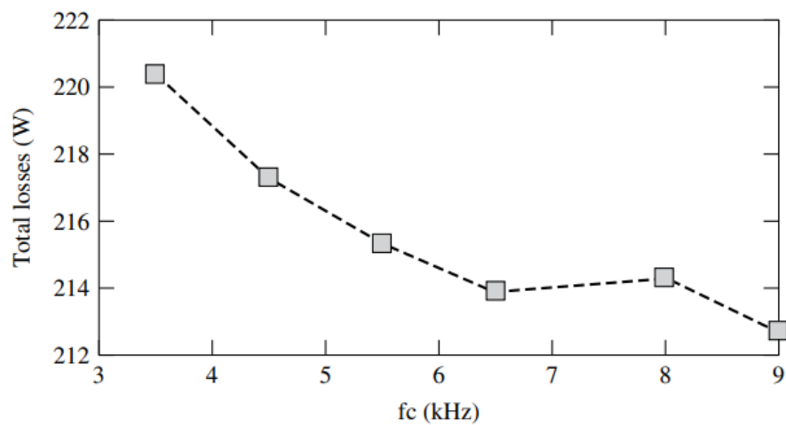
Gambar 10.17 Rugi pada frekuensi switching yang berbeda.
