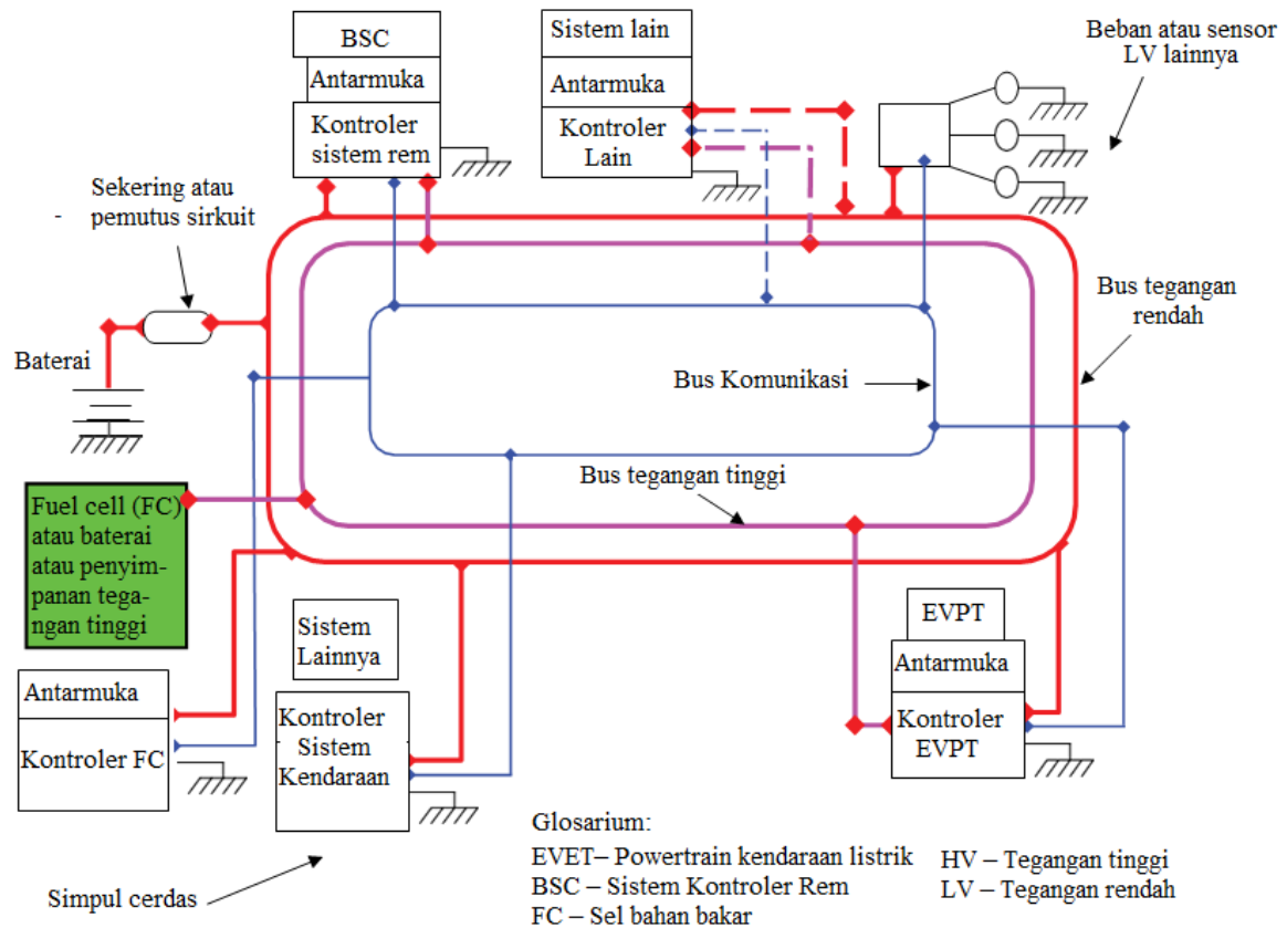
Gambar 2.6 Diagram susunan sistem dari EV. Dari © 2008 IEEE.
