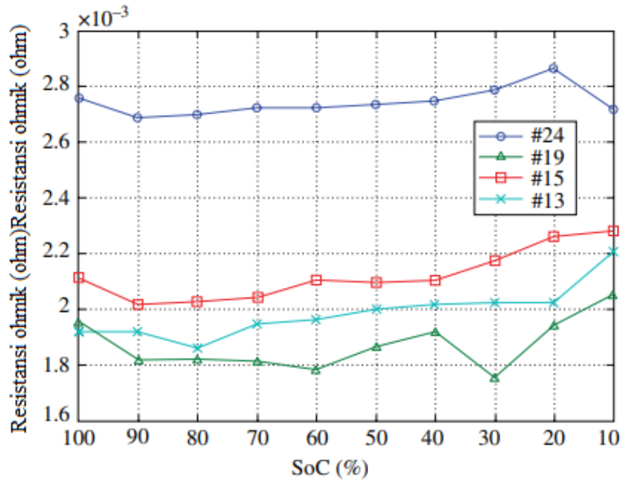
Gambar 12.7 Hasil Identifikasi Resistansi Ohmik Rt.
