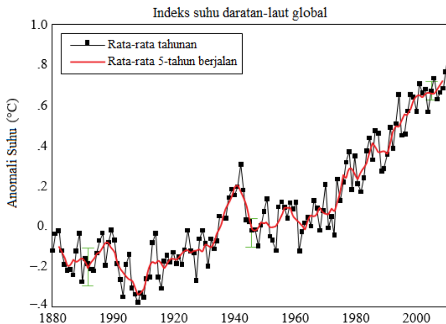
Gambar 1.6 Perubahan suhu udara permukaan rata-rata tahunan global.
