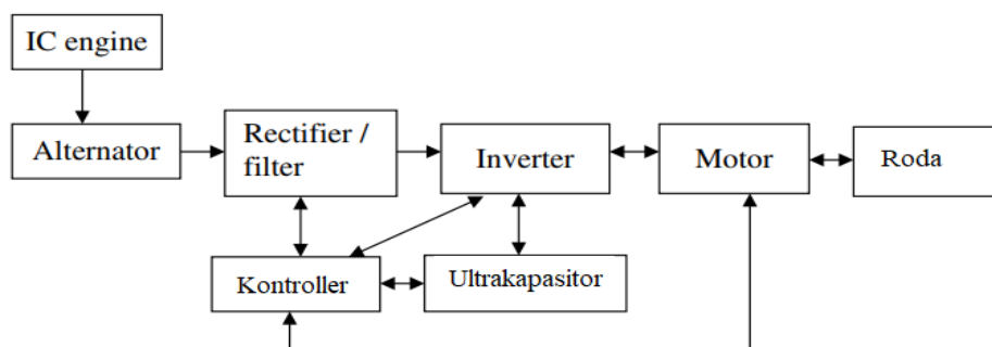
Gambar 6.8 Arsitektur taraf sistem menurut sistem kendaraan off-road hybrid menggunakan ultrakapasitor buat penyimpanan.
