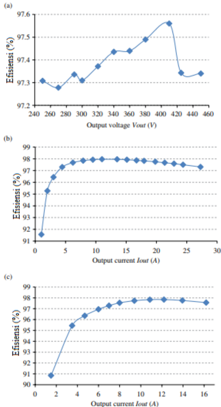
Gambar 13.13 Kinerja prototipe konverter LLC: (a) Efisiensi terukur vs tegangan output pada P_o = 6,6 kW dan V_{in} = 390 V. (b) Efisiensi terukur vs arus output pada V_o = 250 V dan V_{in} = 390 V. (c) Efisiensi terukur vs arus output pada V_o = 410 V dan V_{in} = 390 V.
