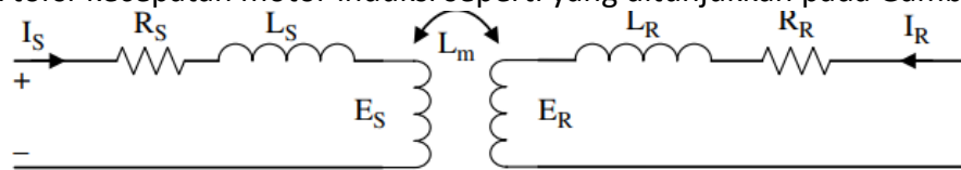
Gambar 10.3 Rangkaian stator dan rotor mesin induksi.
