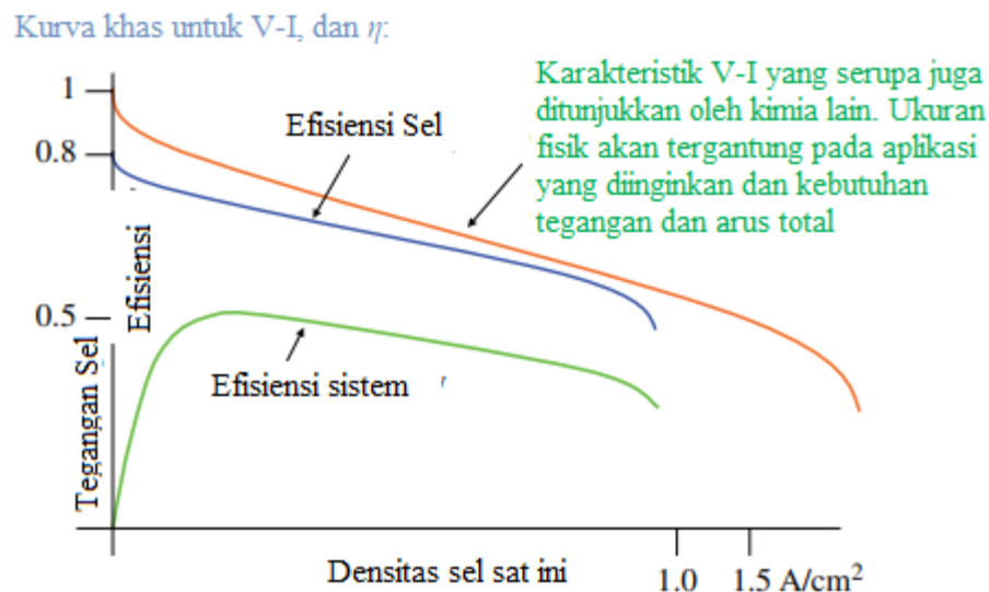
Gambar 11.27 Karakteristik sel bahan bakar.
