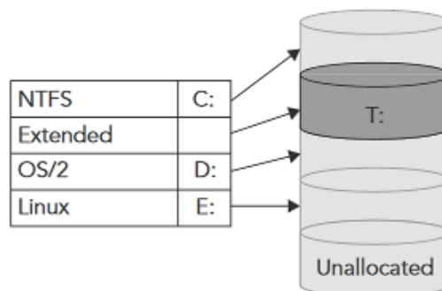
Gambar 7.10 Disk Drive dengan Extended Partition
