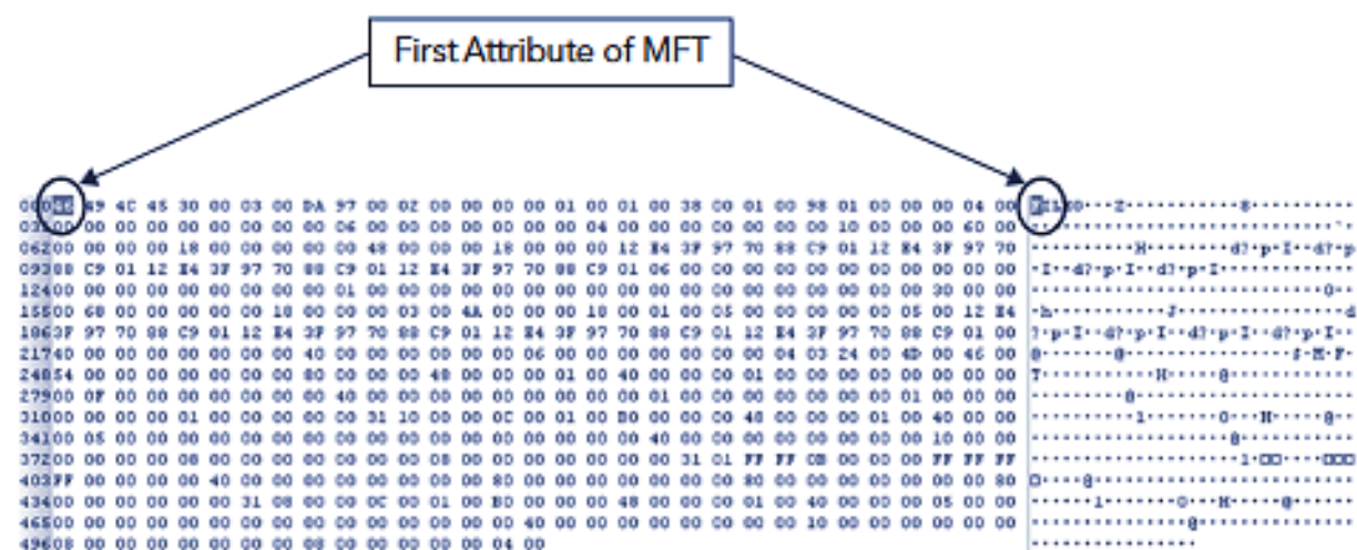
Gambar 9.4 Entri Atribut Pertama di Sektor Pertama MFT
