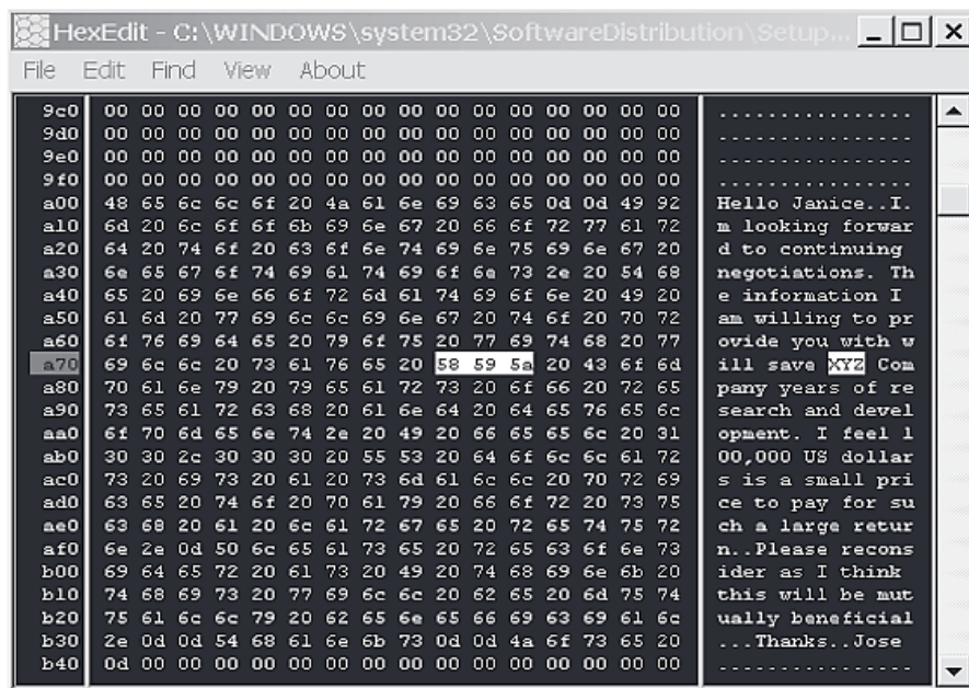
Gambar 4.17 Identifikasi HEX dan ASCII Perusahaan “XYZ”.
