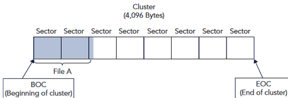
Gambar 8.1 Pemanfaatan Sektor dari File yang Disimpan dalam Cluster
