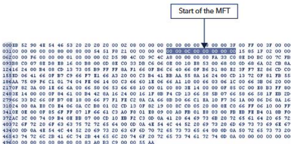
Gambar 9.3 Byte Offset 48 sampai 55 dan Awal dari MFT
