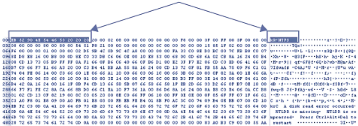
Gambar 9.1 Sektor Pertama dari Boot Record (NTFS)
