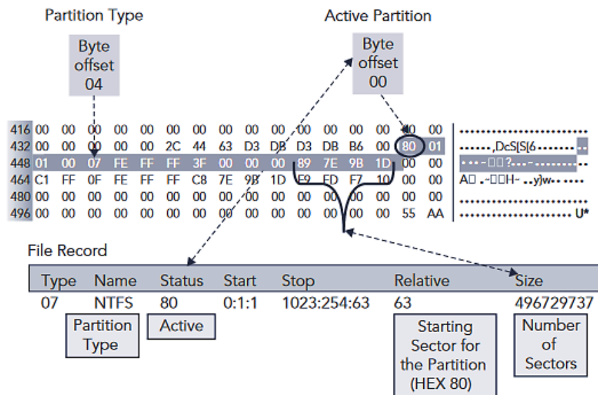
Gambar 7.4 Tabel Partisi yang Terkandung dalam MBR
