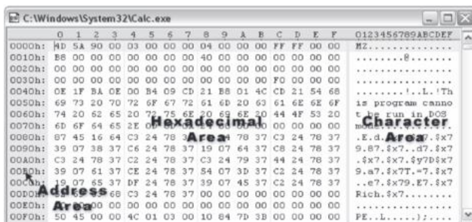
Gambar 5.11 Tata Letak Editor HEX Umum
