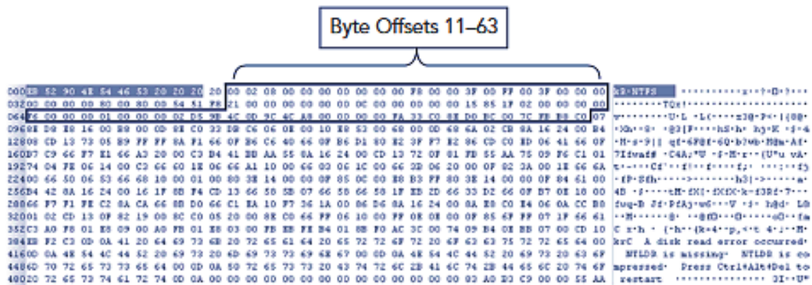
Gambar 9.2 Offset Byte 11 sampai 63 Berisi Informasi Parameter Partisi
