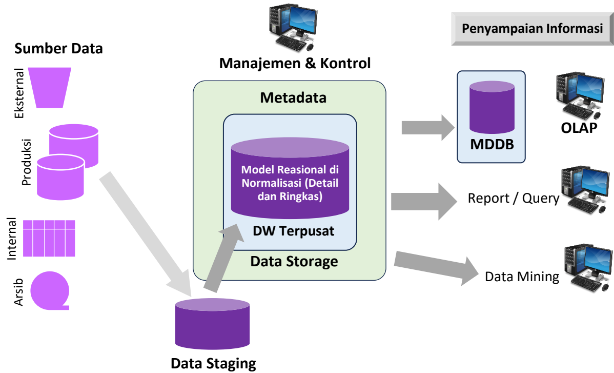
Gambar 7.7 Ikhtisar komponen gudang data terpusat.
