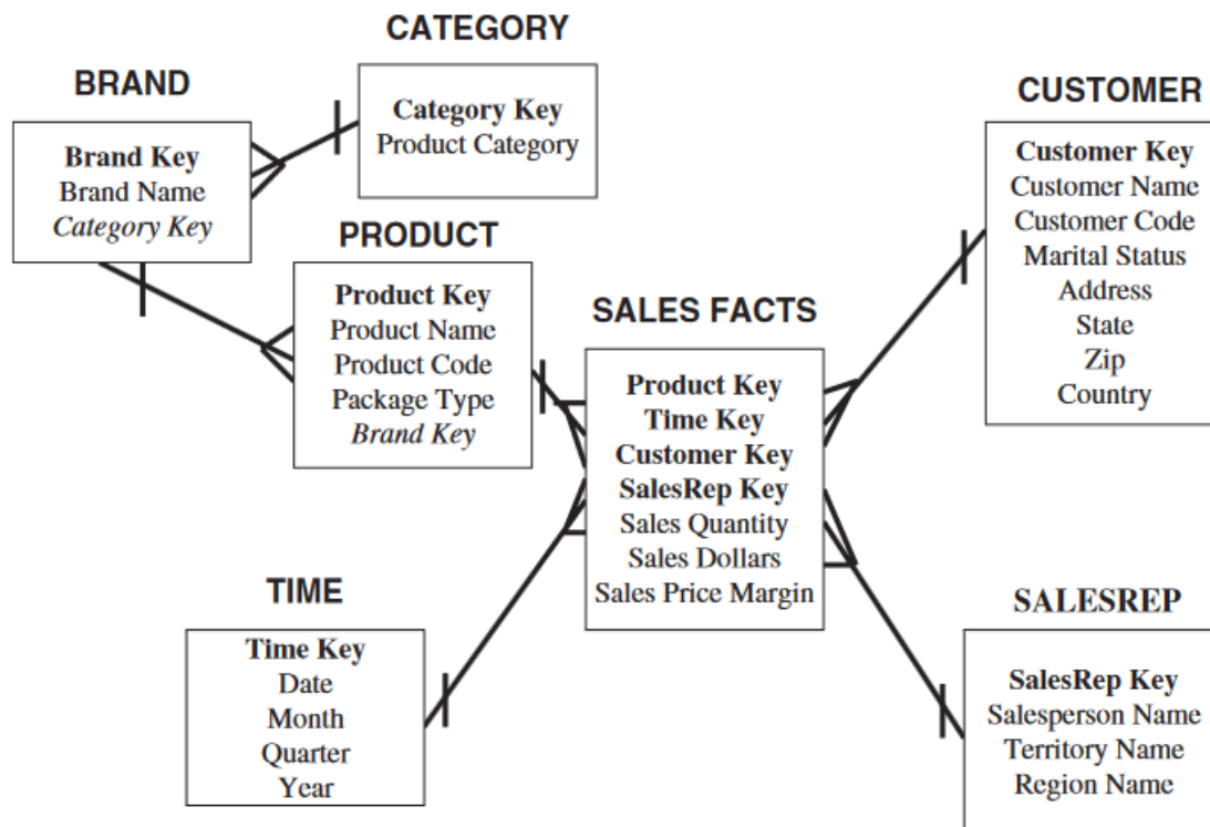
Gambar 11.8 Dimensi produk: dinormalisasi sebagian.
