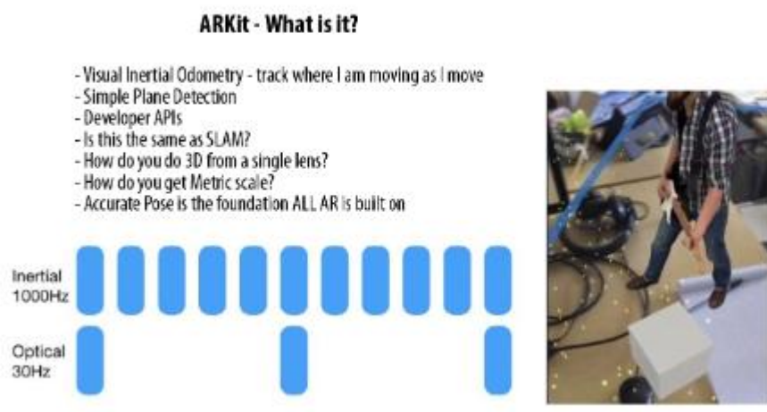
Gambar 5.20. ARKit Apple
