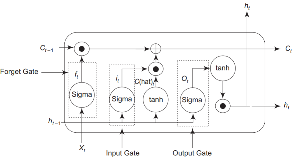
Gambar 16.4 Struktur CNN-LSTM.
