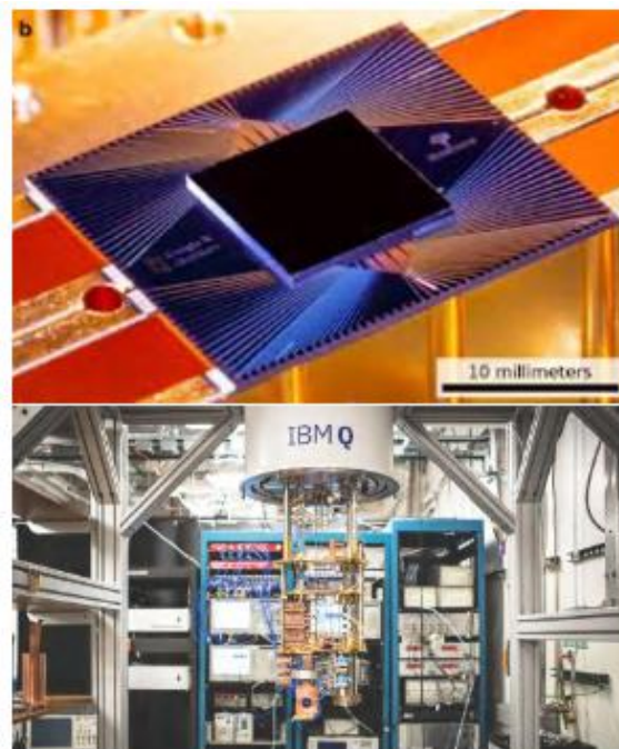
Gambar 2.3 Cip Sycamore milik Google (atas) dan perangkat pendingin komputer kuantum superkonduktor IBM (bawah). Gambar diambil dari https://www.nature.com/articles/s41586-019-1666-5 (atas) dan https://www.ibm.com/quantum (bawah).
