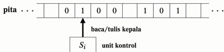
Gambar 2.1 Gambar skematis mesin Turing, yang memperlihatkan pita, kepala baca/tulis, dan unit kendali.
