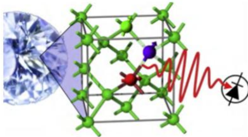
Gambar. 4.1 Pusat warna pada intan, yang terbentuk akibat adanya cacat (atom nitrogen, berwarna merah pada gambar) dan kekosongan di sebelahnya (berwarna biru pada gambar) dalam struktur kristal intan, yang hampir seluruhnya tersusun dari atom karbon. Pusat warna ini digunakan sebagai sensor. Gambar diambil dari
