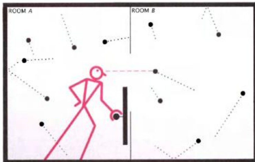
Gambar 3.7 Gambar skematis paradoks iblis Maxwell. Iblis tersebut, dengan membuka dan menutup pintu kecil, memisahkan molekul-molekul yang lebih cepat dari yang lebih lambat. Gambar diambil dari https://www.jstor.org/stable/24979551 .
