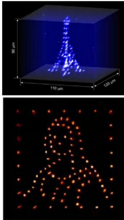
Gambar 2.4 Atom Rydberg dalam konfigurasi artistik yang diperoleh dengan memosisikan atom-atom tersebut (titik-titik dalam gambar) menggunakan pinset optik. Gambar diambil dari https://www.usinenouvelle.com/article/calcul-quantique-pasqal-s-impose-dans-la-cour-des-grands-avec-ses-atomes-froids.N1809802 (atas) dan dari https://journals.aps.org/pr/abstract/10.1103/PhysRevA.102.063107 (bawah).
