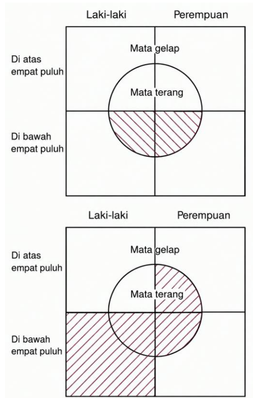
Gambar 1.6 Contoh ketidaksamaan Bell dalam kehidupan sehari-hari.
