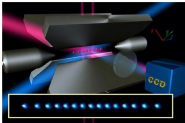
Gambar 2.2 Ion yang terperangkap (diperbesar di bagian bawah) oleh medan listrik (pelat dan ujung runcing pada gambar). Manipulasi dan pengukuran (pengukuran dilakukan melalui kamera khusus yang disebut CCD) terhadap keadaan ion dilakukan dengan memancarkan cahaya laser (atas izin Rainer Blatt, Universitas Innsbruck).
