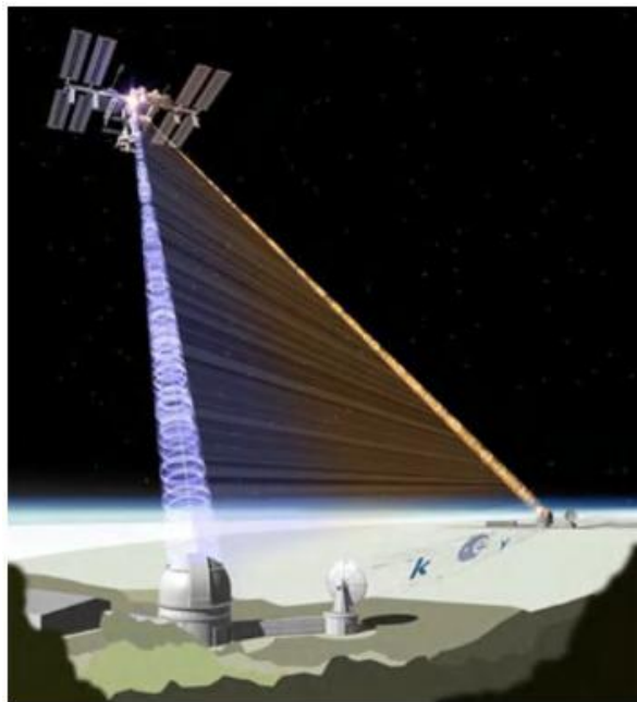
Gambar 3.6 Ilustrasi skematis distribusi keterikatan ( entanglement ) melalui satelit. Pasangan foton yang terikat didistribusikan ke dua lokasi di Bumi yang terpisah jarak ribuan kilometer.
