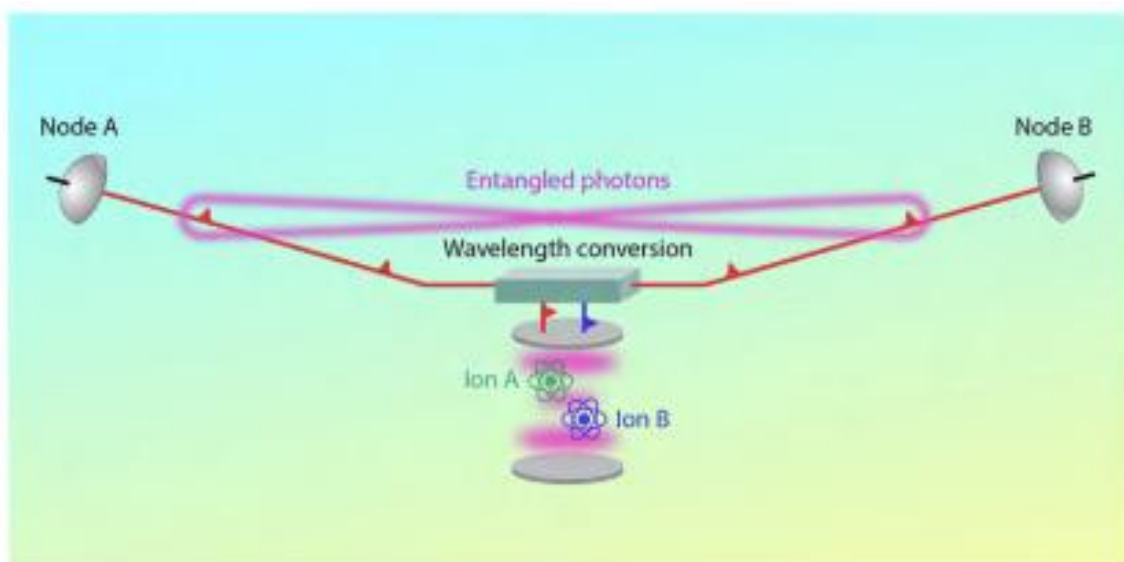
Gambar 3.5 Skema pengulang kuantum (Gambar diambil dari https://physics.aps.org/articles/v16/84 ). Keterikatan ( entanglement ) antara ion A dan foton yang dikirim ke simpul A (berjarak 25 kilometer) serta antara ion B dan foton yang dikirim ke simpul B (berjarak 25 kilometer) diubah menjadi keterikatan antara kedua foton tersebut (yang terpisah sejauh 50 kilometer).
