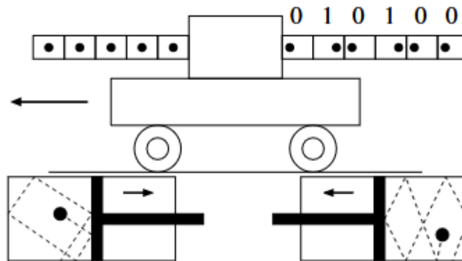
Gambar. 3.8 Pemanfaatan informasi untuk menghasilkan kerja. Informasi yang masuk (nilai bit 0 atau 1 yang merepresentasikan posisi kiri atau kanan molekul di dalam kotak) hilang pada tahap keluaran.
